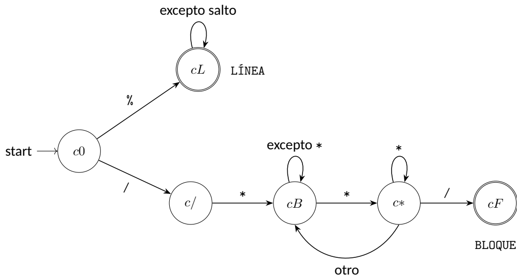
Figura 5: Autómata para comentarios de línea y de bloque.
