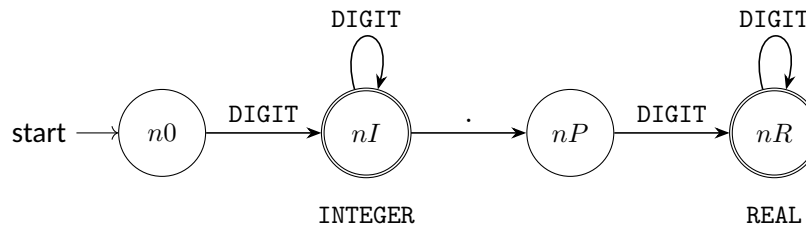
Figura 3: Autómata para números enteros y reales.
