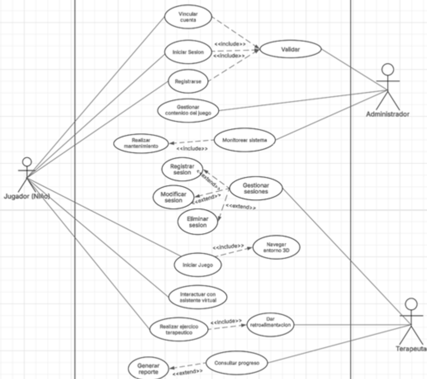
Diagrama de Casos de Uso sobre el funcionamiento de la aplicación TICO AI
