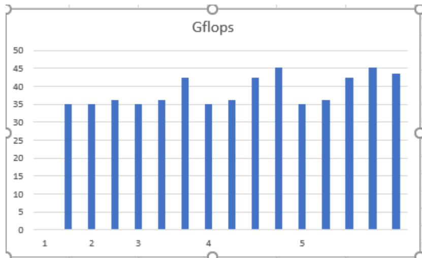
Ilustración 7 Grafica Gflops
