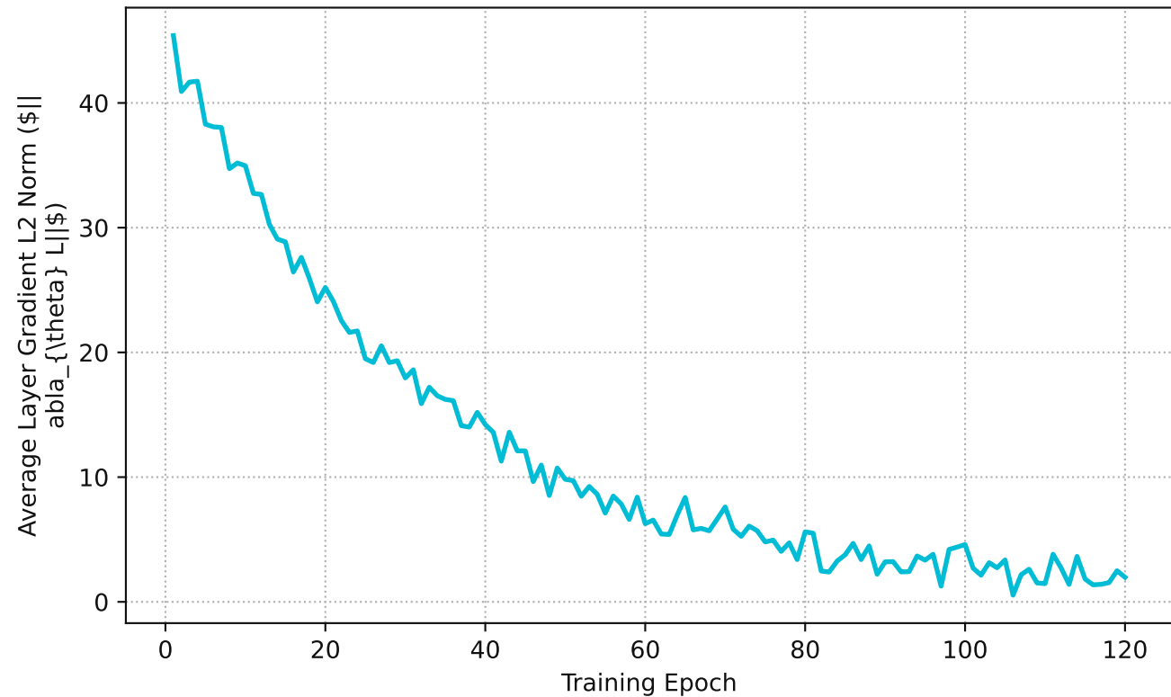
Gradient Norm Convergence
