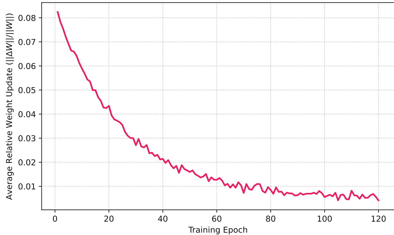
Parameter Update Magnitude Profile
