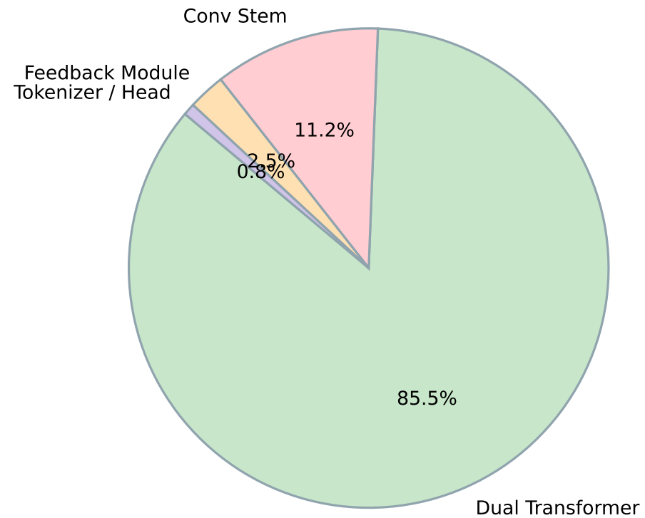
FLOPs Percentage per Module
