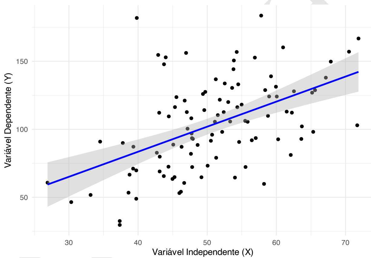
Figura 30.3: Regressão linear.
