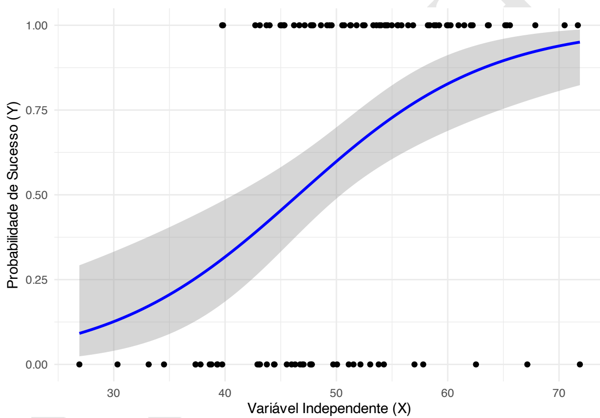
Figura 38.2: Regressão logística.
