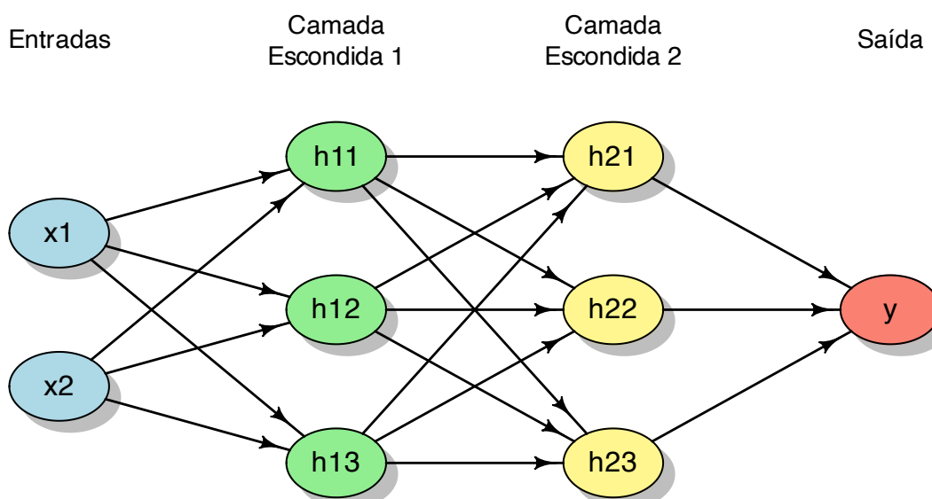
Figura 39.6: Representação esquemática de uma rede neural multicamadas com 2 camadas escondidas além das camadas de entrada e saída.
