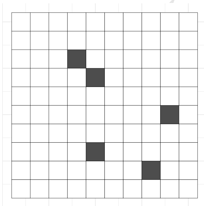
Figura 44.1: Visualização espacial de p < 0,05 (5 quadrados aleatórios em 100).
