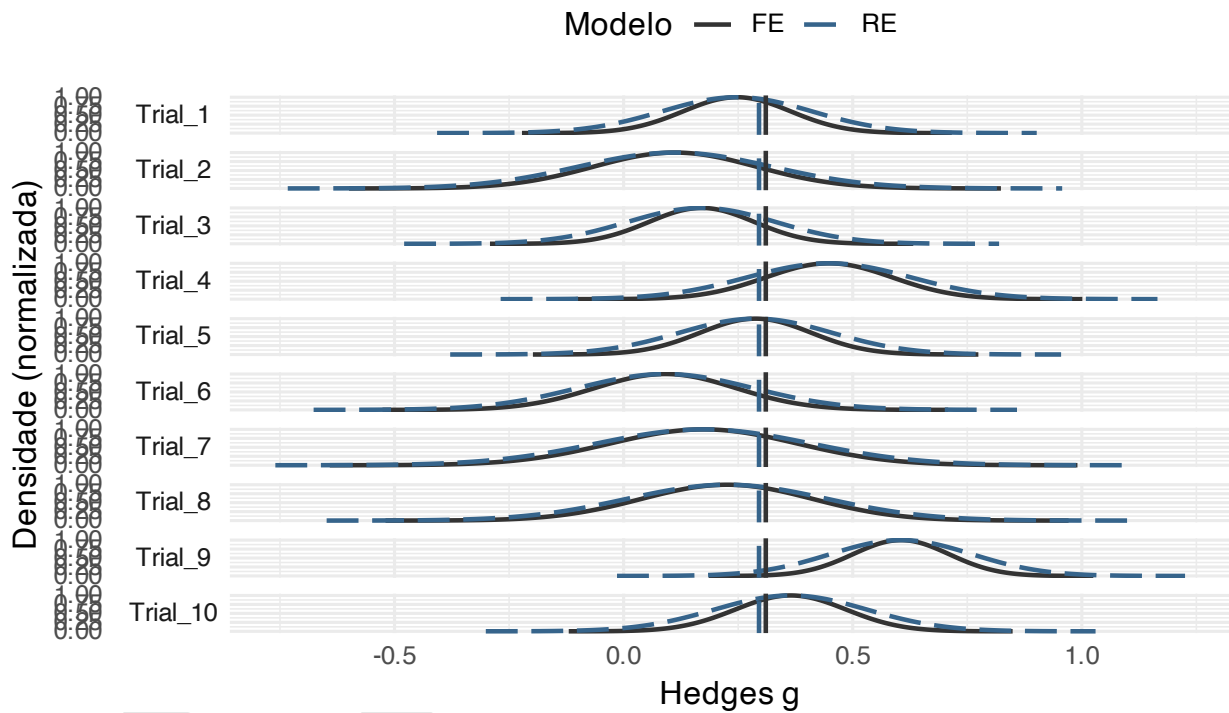
Figura 73.1: Comparação entre modelos de efeito fixo e aleatório com 10 ensaios clínicos simulados.
