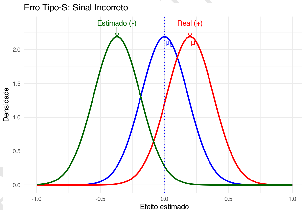
Figura 42.9: Representação gráfica do erro tipo S (sinal) em um teste de hipótese (bicaudal).
