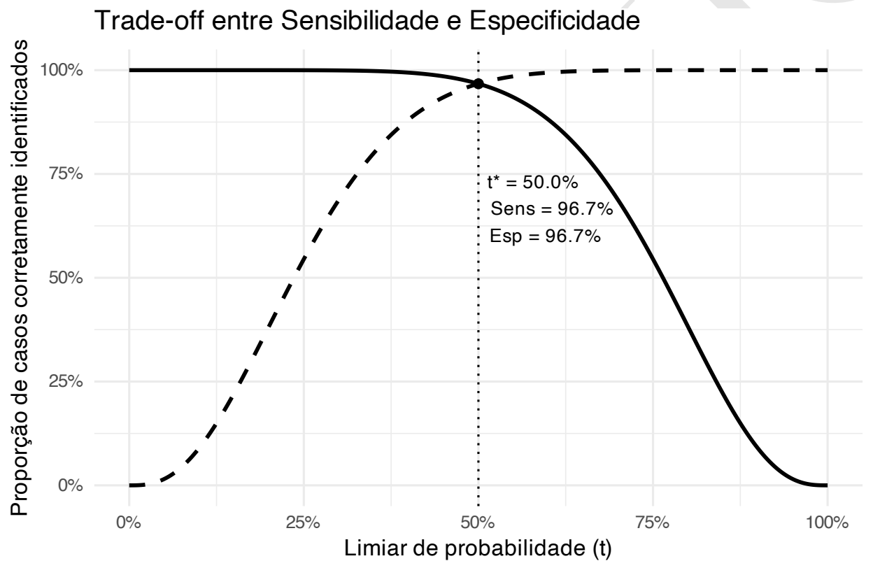
Figura 64.2: Trade-off entre sensibilidade e especificidade em função do limiar de probabilidade (t) para um modelo de classificação.
