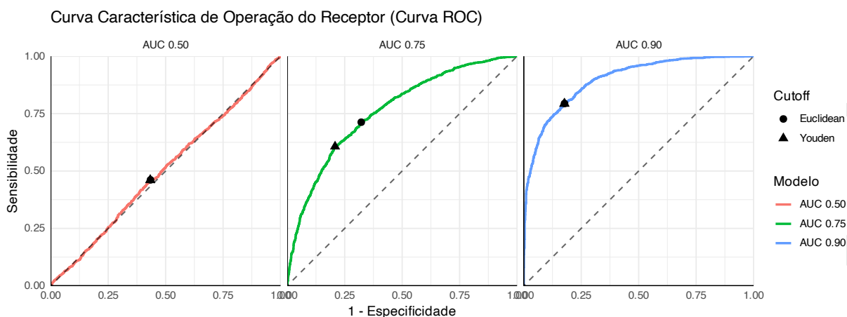
Figura 64.3: Curva ROC (Receiver Operating Characteristic) para um modelos de classificação com diferentes desempenhos diagnósticos.
