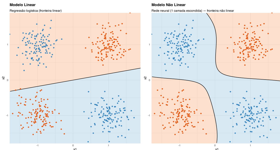
Figura 40.5: Comparação do espaço de decisão entre um modelo linear (regressão logística) e um modelo não linear (MLP).
