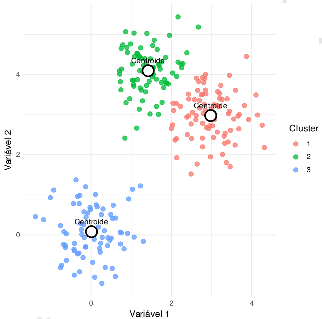
Figura 39.6: Aplicação do algoritmo k-means para identificar grupos em um conjunto de dados bidimensional.
