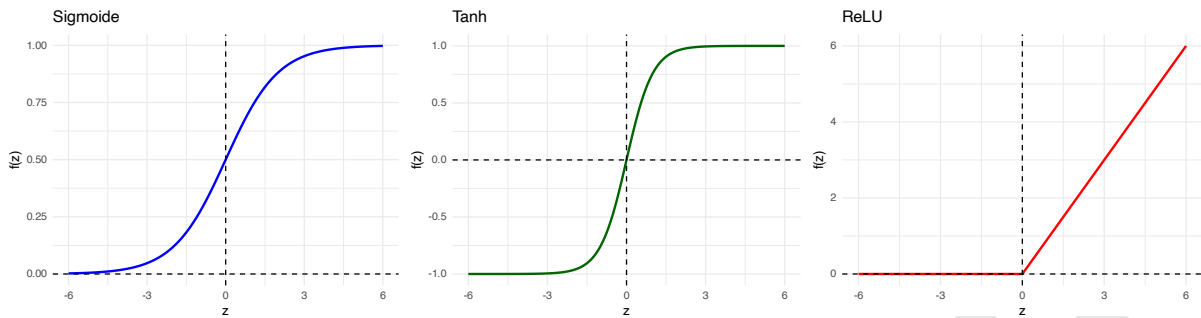
Figura 40.3: Gráficos das funções de ativação mais comuns.
