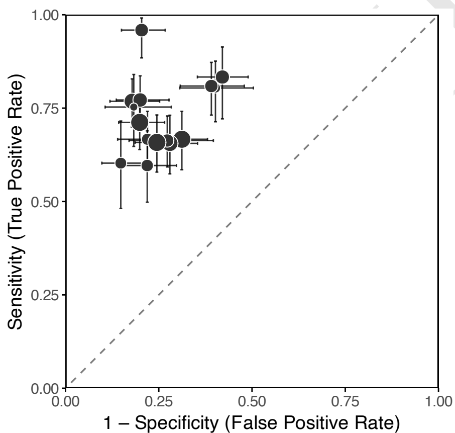
Figura 73.5: Gráfico de cruces em espaço de curva característica de operação do receptor (ROC) para 15 estudos simulados de desempenho diagnóstico.
