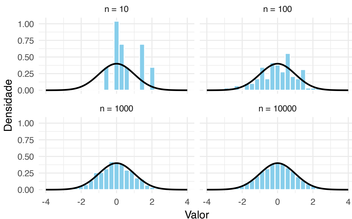
Figura 69.2: Convergência do histograma para a PDF teórica da Normal(0,1) com o aumento do tamanho amostral ( n = 10, 100, 1000, 10000 ).
