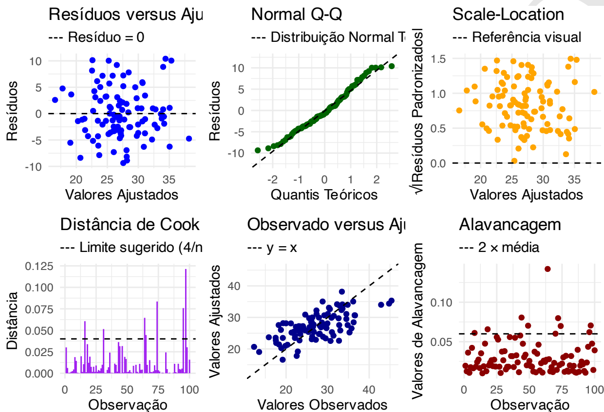
Figura 41.1: Diagnóstico de regressão para avaliar suposições do modelo: linearidade, normalidade dos resíduos, homoscedasticidade e alavancagem.
