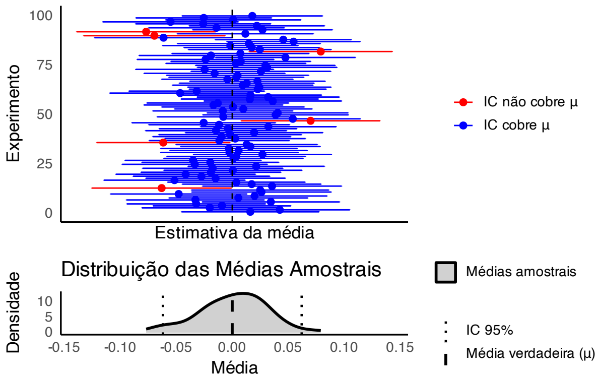
Figura 42.5: Simulação ilustrativa de intervalos de confiança (IC) em 100 experimentos independentes, cada um com 1.000 observações amostradas de uma população normal padrão (média = 0, desvio-padrão = 1). Os ICs são construídos no nível de 95%. O gráfico superior mostra os ICs individuais para cada experimento, indicando se o IC cobre ou não a média verdadeira ( \mu = 0 ). O gráfico inferior apresenta a distribuição das médias amostrais obtidas nos experimentos, juntamente com o IC teórico para a média populacional. Observe que aproximadamente 95% dos ICs individuais cobrem a média verdadeira, ilustrando o conceito de cobertura no longo prazo associado aos intervalos de confiança.
