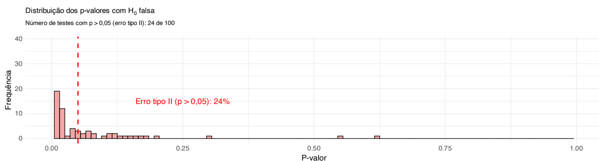
Figura 42.8: Erro tipo II: Distribuição dos p-valores em 100 testes de hipótese de amostras aleatórias de tamanho 10. A linha vermelha pontilhada indica o nível de significância estatística de 0,05.
