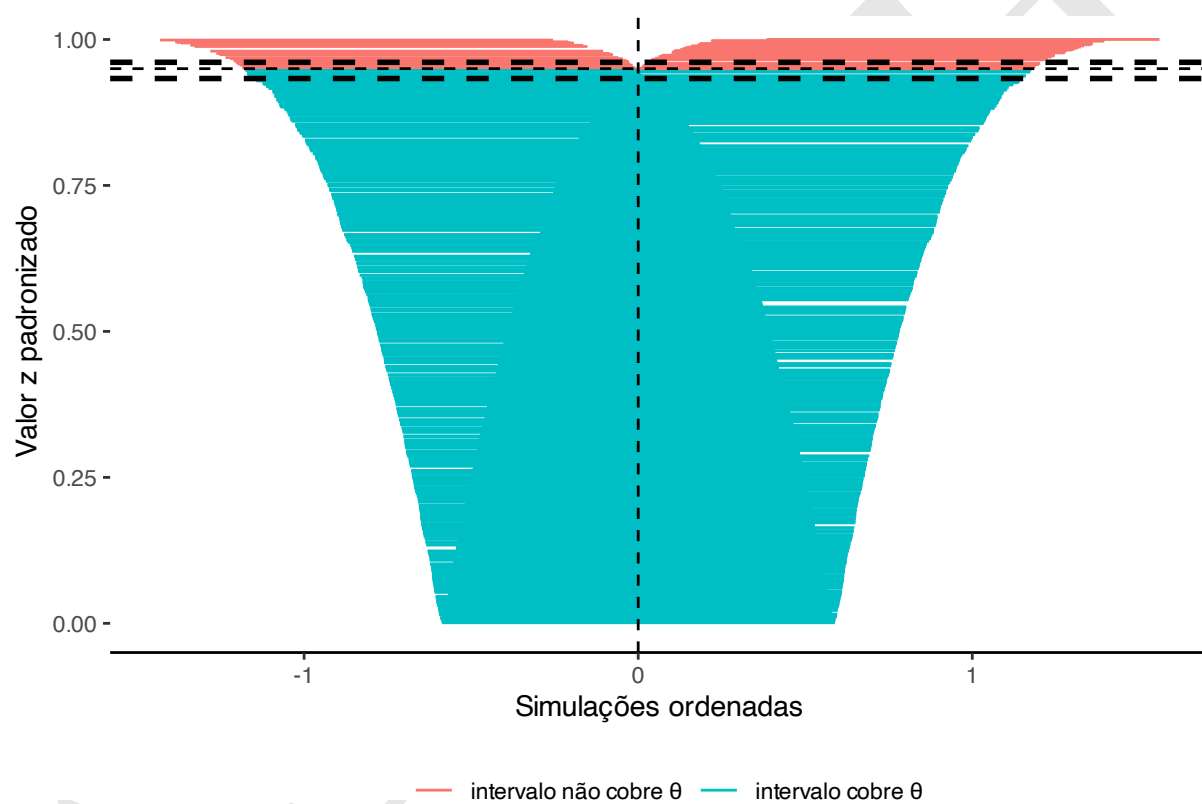
Figura 69.4: Cobertura de Intervalos de Confiança em um estudo de simulação.
