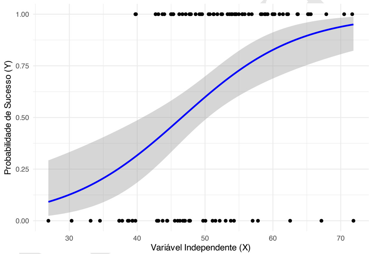
Figura 39.2: Regressão logística.
