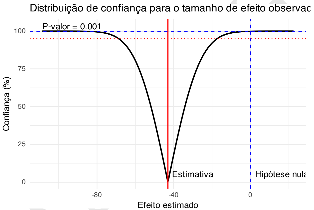
Figura 45.2: Distribuição de confiança para o tamanho de efeito estimado.
