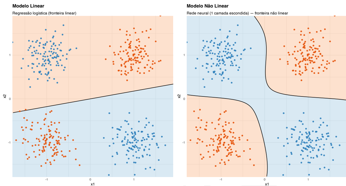
Figura 41.5: Comparação do espaço de decisão entre um modelo linear (regressão logística) e um modelo não linear (MLP).
