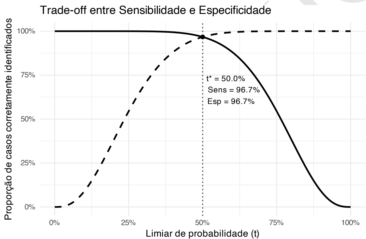
Figura 63.2: Trade-off entre sensibilidade e especificidade em função do limiar de probabilidade (t) para um modelo de classificação.
