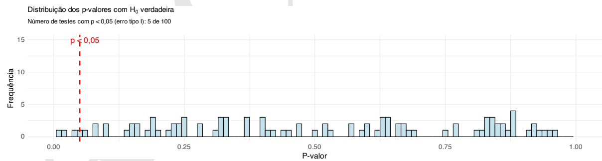
Figura 41.7: Erro tipo I: Distribuição dos p-valores em 100 testes de hipótese de amostras aleatórias de tamanho 30. A linha vermelha pontilhada indica o nível de significância estatística de 0,05.
