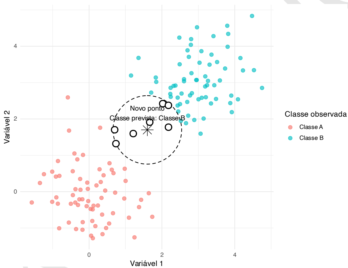
Figura 38.3: Classificação usando o algoritmo KNN.
