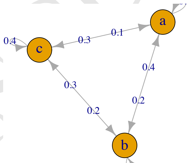
Figura 36.1: Cadeia de Markov com 3 estados (a, b, c) e suas probabilidades de transição.
