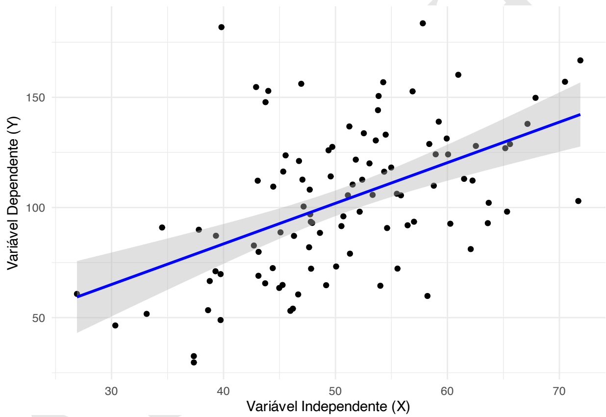
Figura 30.3: Regressão linear.
