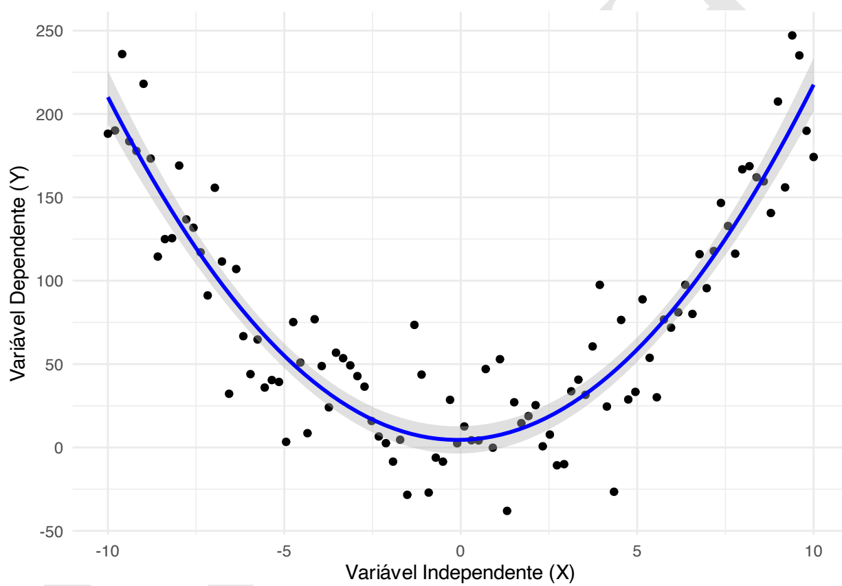
Figura 30.5: Regressão não-linear.
