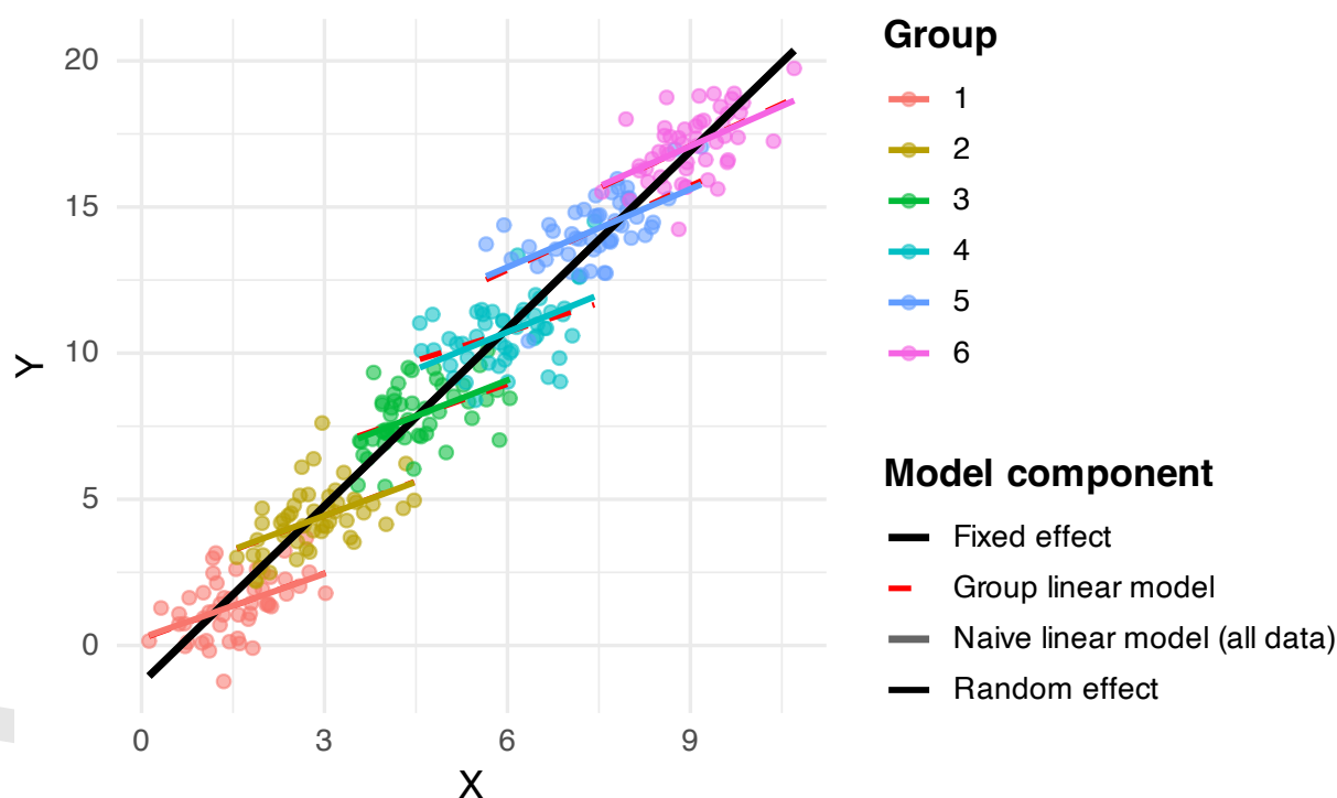
Figura 31.11: Efeitos fixos, aleatórios e mistos em dados simulados com paradoxo de Simpson. As linhas vermelhas representam os efeitos dentro dos grupos, enquanto as linhas cinza e preta representam os efeitos globais. O modelo misto (linhas coloridas) captura os efeitos dentro dos grupos.
