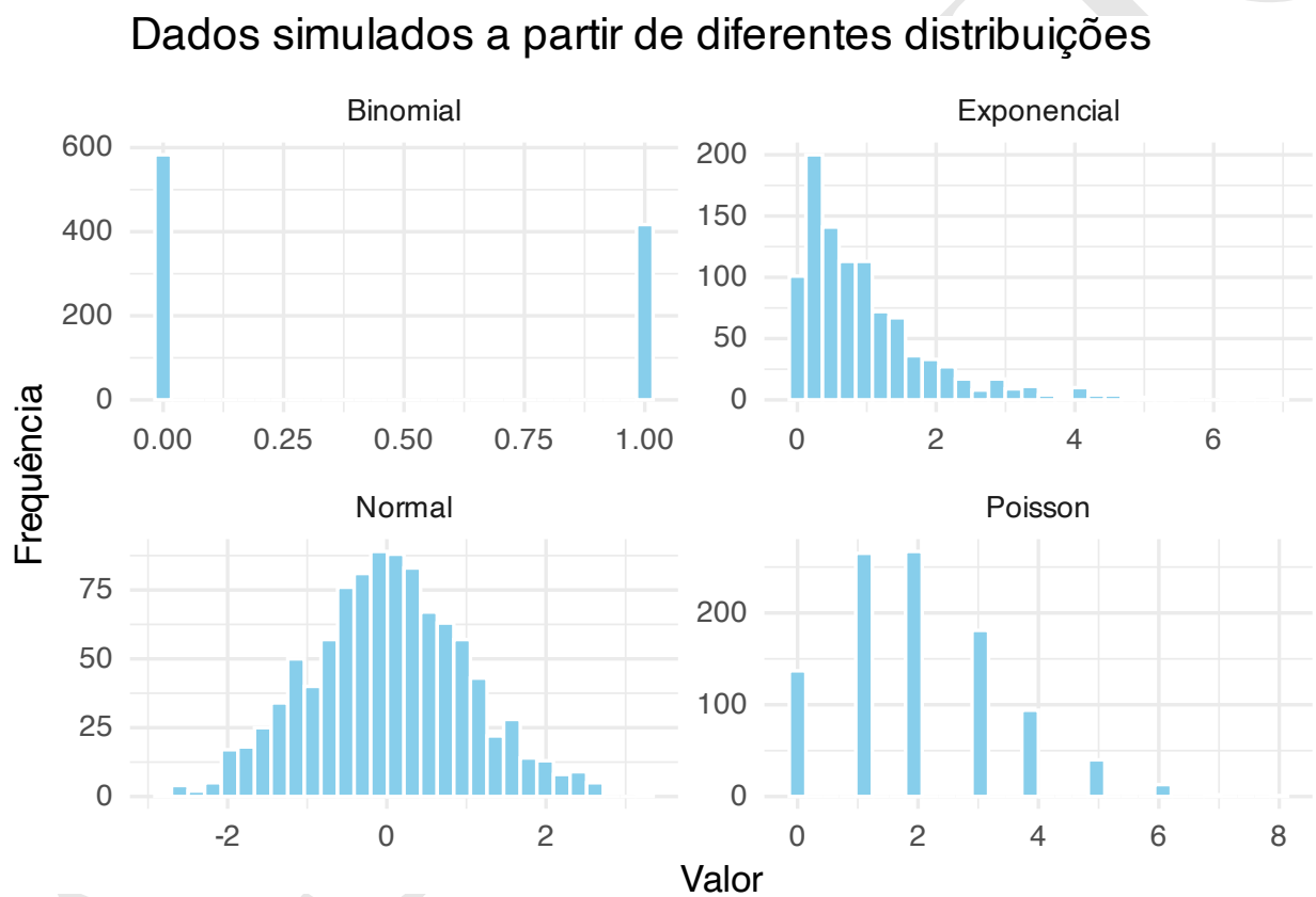
Figura 70.1: Dados simulados a partir de diferentes distribuições: Normal(0,1), Binomial(1,0.4), Poisson(2) e Exponencial(1).
