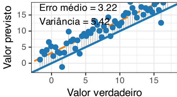
Alto Viés / Alta Variância
