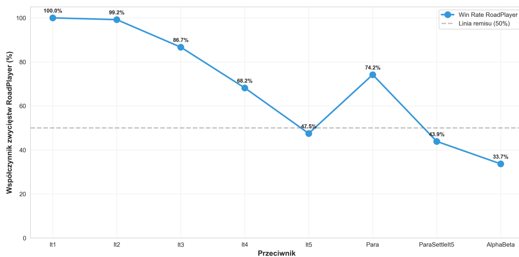
Rysunek 8.18: Skuteczność RoadPlayer w zależności od jakości przeciwnika
