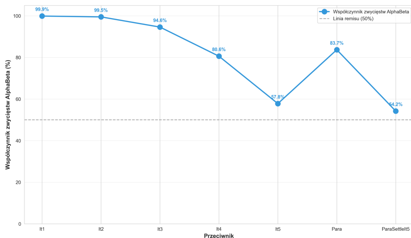
Rysunek 8.6: Skuteczność AlphaBetaPlayer w zależności od jakości przeciwnika
