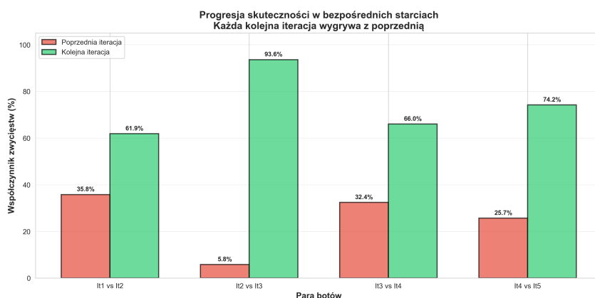
Rysunek 8.4: Porównanie wyników par botów w scenariuszu 2
