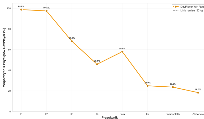
Rysunek 8.13: Skuteczność DevPlayer w zależności od jakości przeciwnika
