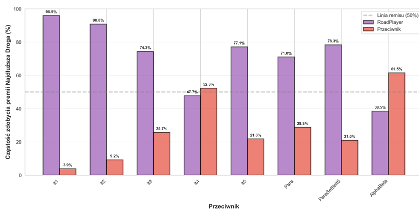
Rysunek 8.17: Częstość zdobycia premii Najdłuższa Droga przez RoadPlayer i przeciwników
