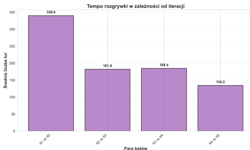
Rysunek 8.5: Porównanie średniej liczby tur w scenariuszu 2
