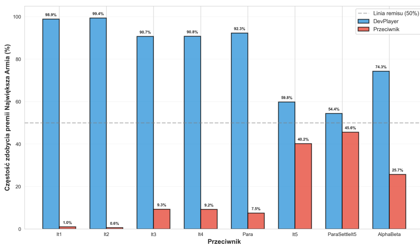
Rysunek 8.15: Częstość zdobycia premii Największa Armia przez DevPlayer i przeciwników
