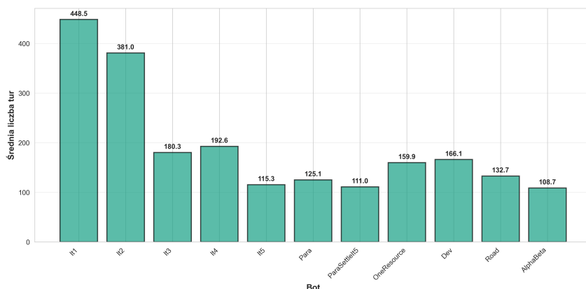
Rysunek 8.2: Zależność tempa rozgrywki od jakości strategii
