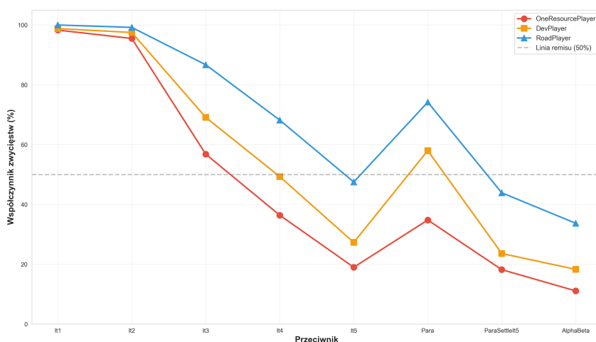
Rysunek 8.18: Porównanie skuteczności strategii wyspecjalizowanych
