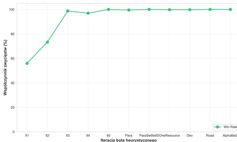
Rysunek 8.1: Skuteczność kolejnych botów przeciwko graczowi losowemu.
