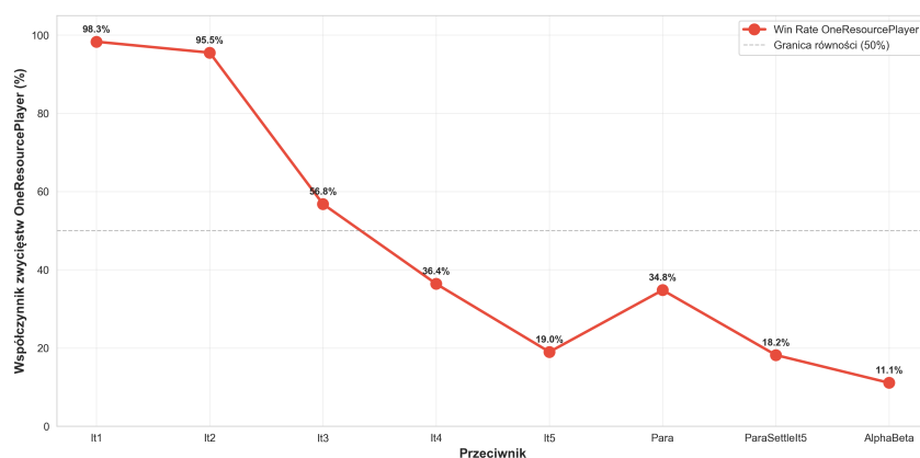
Rysunek 8.12: Skuteczność strategii monosuwrowcowej w zależności od jakości przeciwnika
