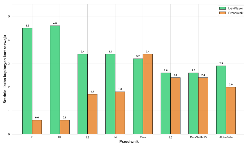
Rysunek 8.14: Średnia liczba kupionych kart rozwoju przez DevPlayer i przeciwników
