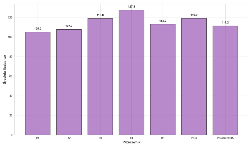
Rysunek 8.7: Tempo rozgrywki AlphaBeta vs różni przeciwnicy
