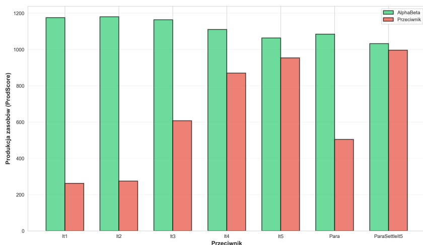
Rysunek 8.10: Porównanie produkcji zasobów AlphaBeta vs przeciwnicy.
