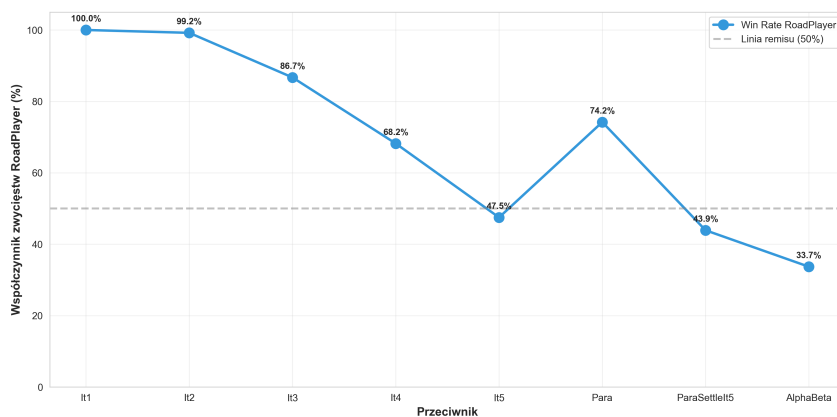
Rysunek 8.16: Skuteczność RoadPlayer w zależności od jakości przeciwnika
