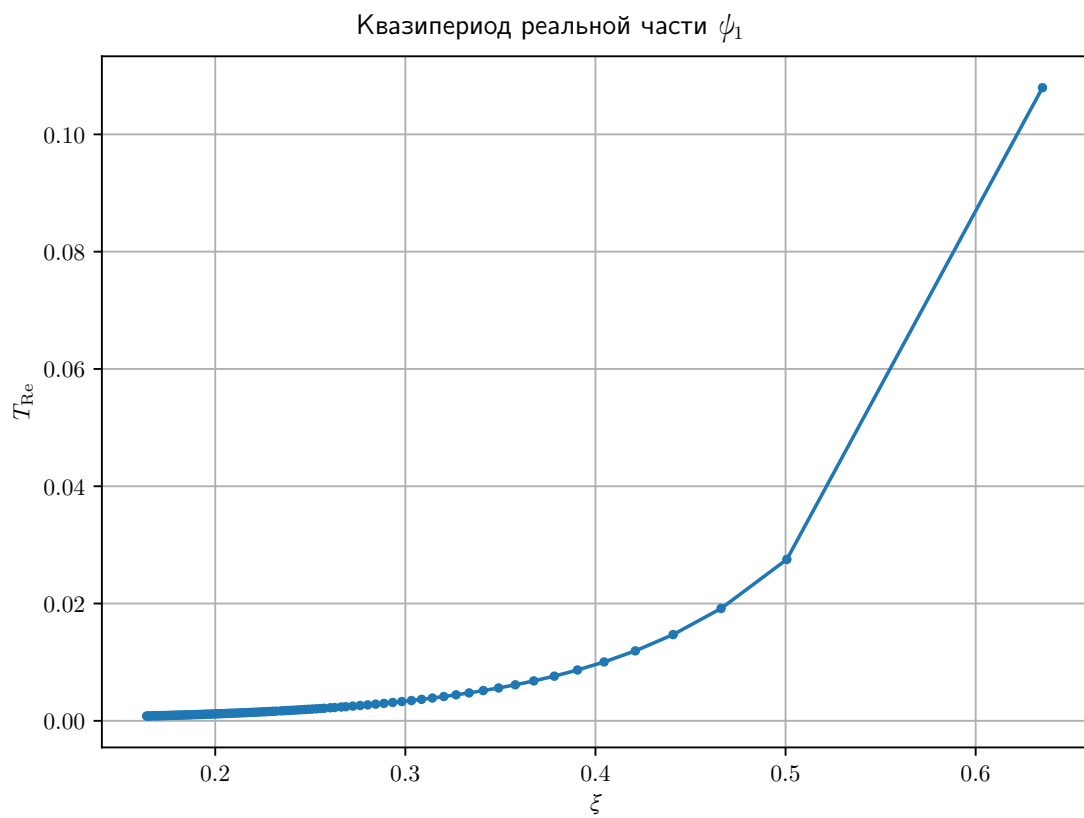
Рис. 13: График зависимости длины квазипериода \text{Re}\Psi_1 от \xi из данных magexр
