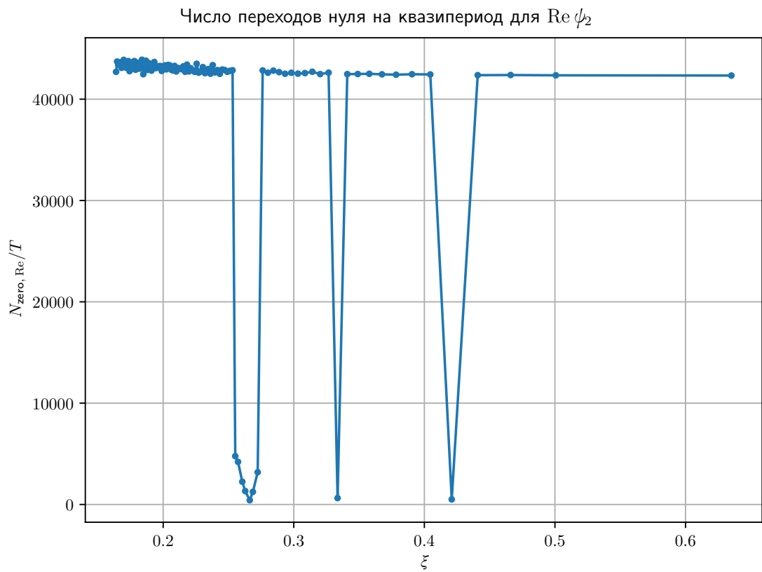
Рис. 19: График количество нулей \text{Re}\Psi_2 на единицу длины квазипериода \Psi_1 из данных magexр
