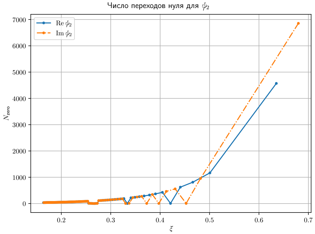
Рис. 11: График количества переходов через ноль Re\Psi_2 и Im\Psi_2 на интервале одного квазипериода \Psi_1 из данных М4
