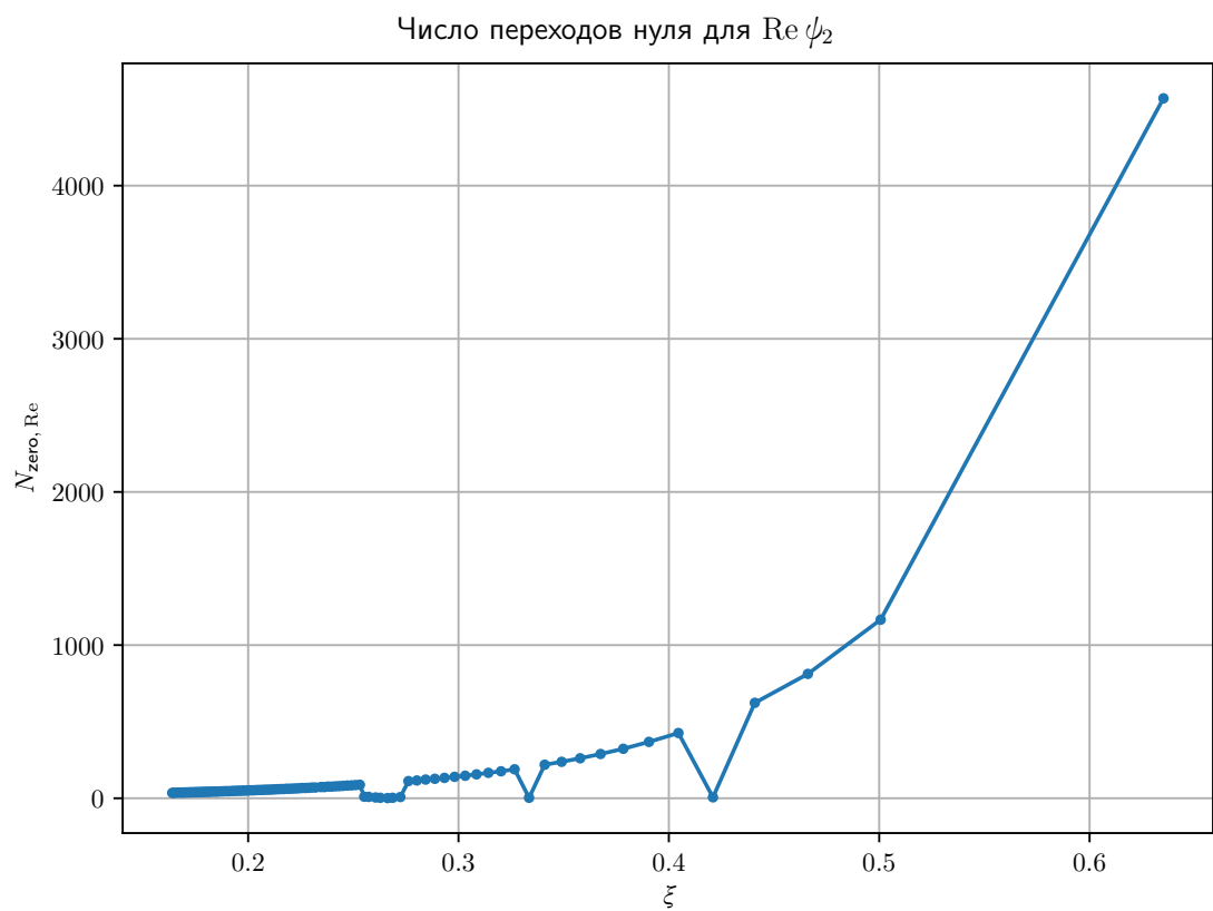
Рис. 15: График количества переходов через ноль \operatorname{Re} \Psi_2 на интервале одного квазипериода \operatorname{Re} \Psi_1 из данных magexr
