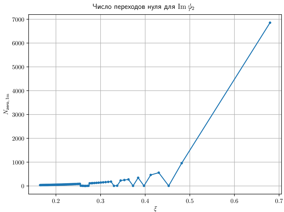
Рис. 16: График количества переходов через ноль \operatorname{Im} \Psi_2 на интервале одного квазипериода \operatorname{Im} \Psi_1 из данных magexr
