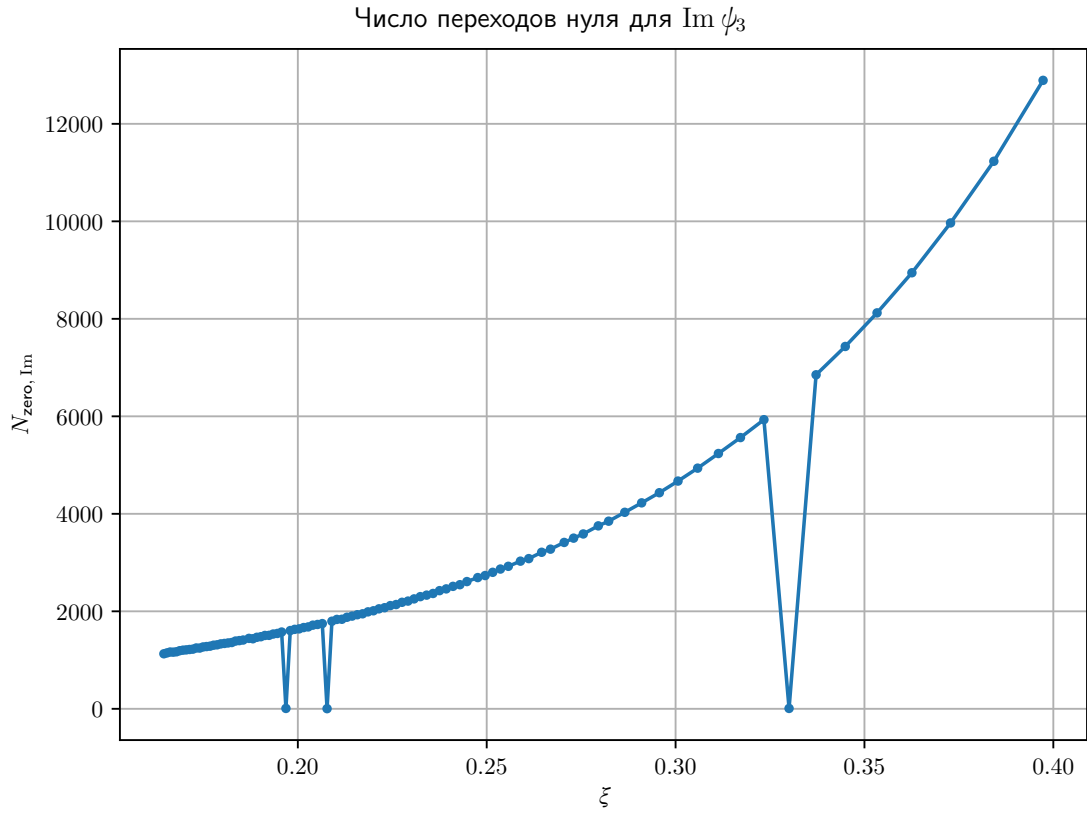
Рис. 18: График количества переходов через ноль \operatorname{Im} \Psi_3 на интервале одного квазипериода \operatorname{Im} \Psi_1 из данных magexr
