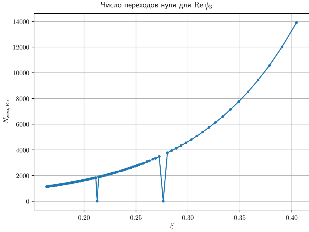
Рис. 17: График количества переходов через ноль \operatorname{Re} \Psi_3 на интервале одного квазипериода \operatorname{Re} \Psi_1 из данных magexr
