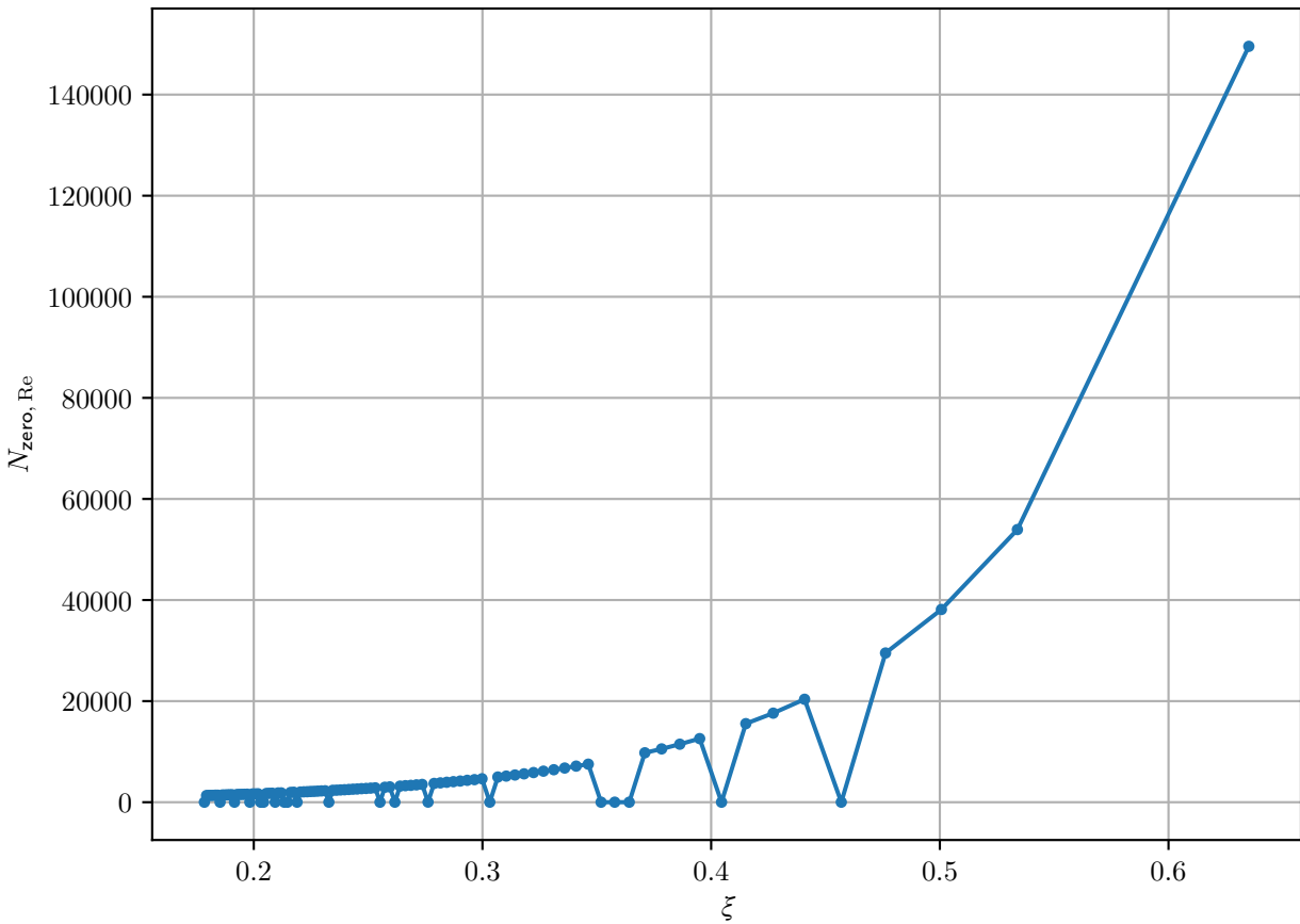
Число переходов нуля для \operatorname{Re} \phi_3
