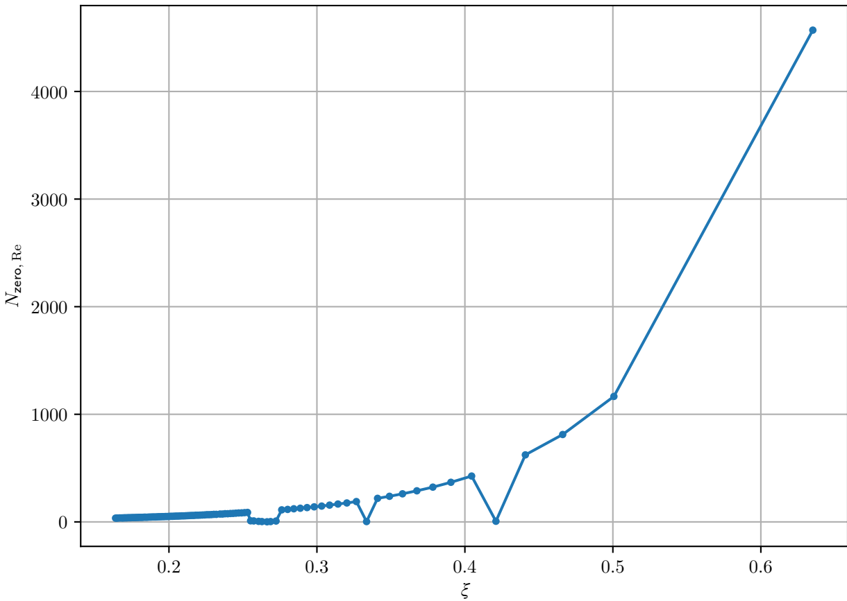
Число переходов нуля для \operatorname{Re} \phi_2
