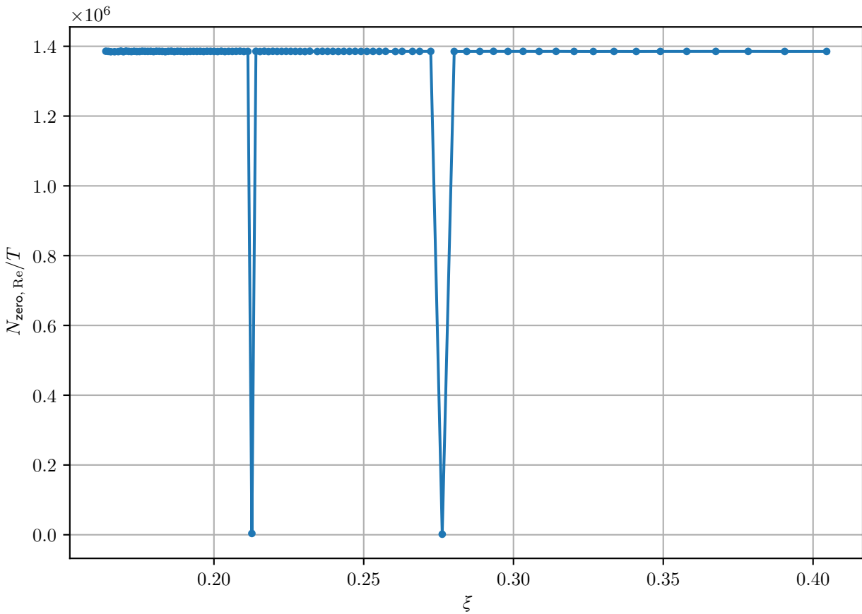
Число переходов нуля на квазипериод для \text{Re } \psi_3
