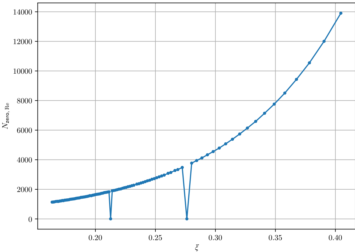
Число переходов нуля для \operatorname{Re} \phi_3
