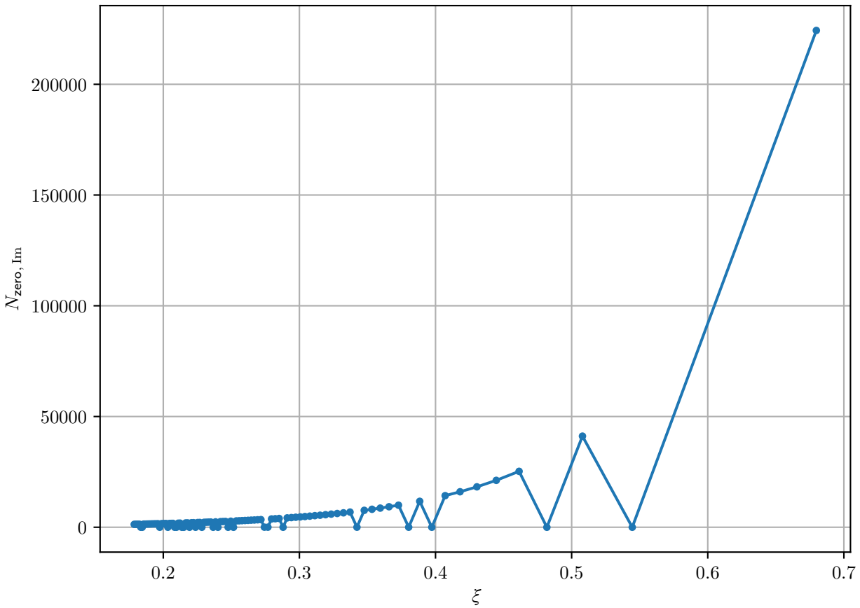
Число переходов нуля для \text{Im } \psi_3
