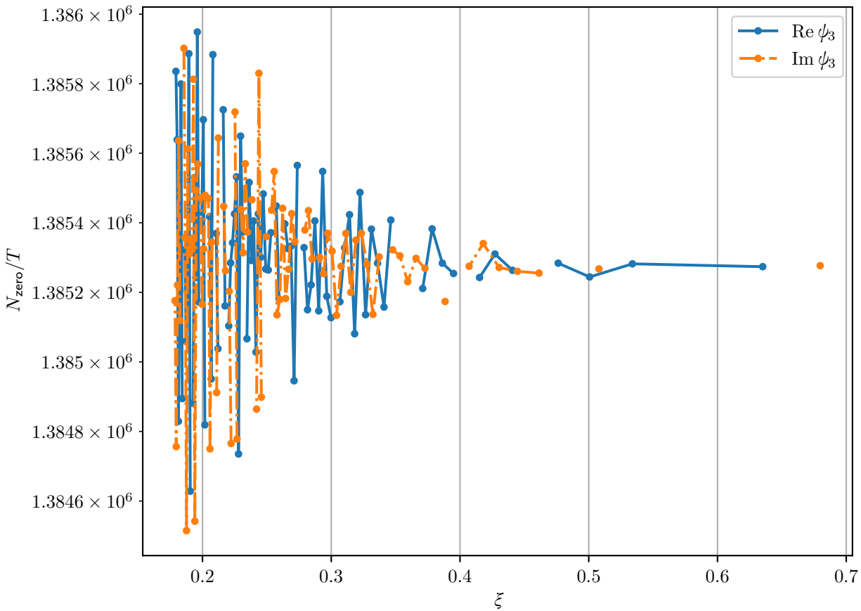
Число переходов нуля на квазипериод для \psi_3
