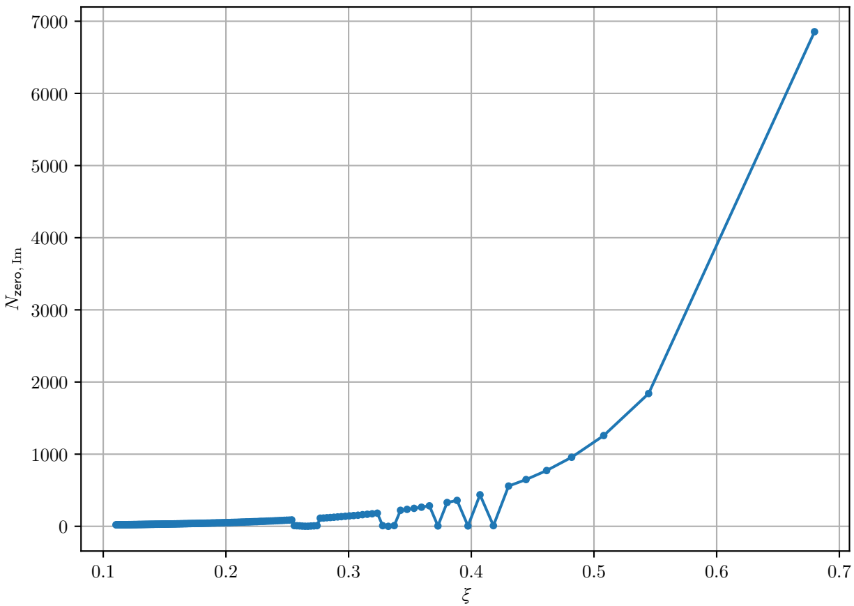
Число переходов нуля для \text{Im } \phi_2
