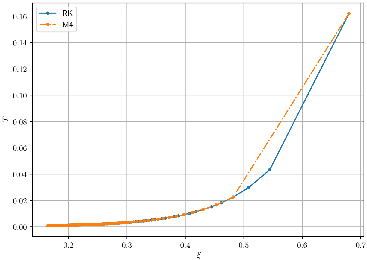
Квазипериод \text{Im } \psi_1 , разные методы
