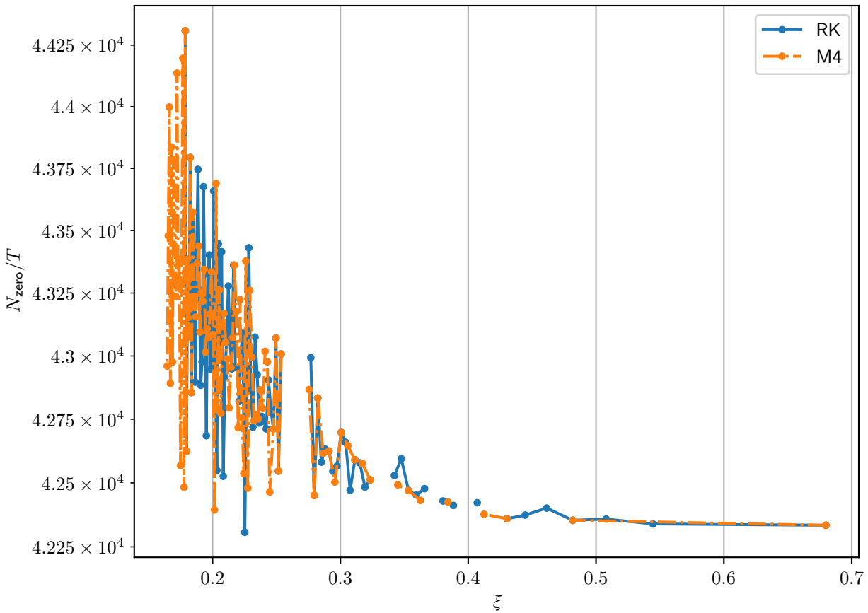
Число переходов нуля на квазипериод для \text{Im } \psi_2 , разные методы
