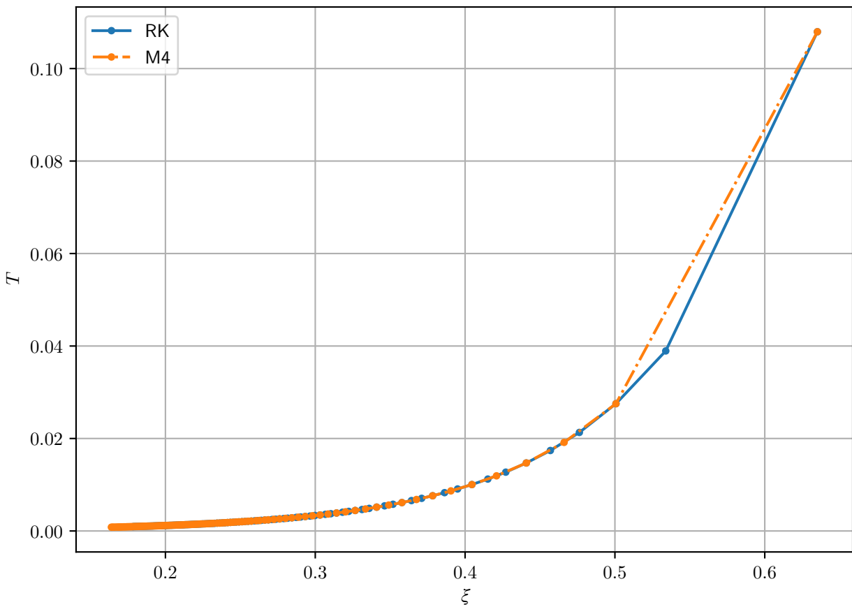
Квазипериод \text{Re } \psi_1 , разные методы
