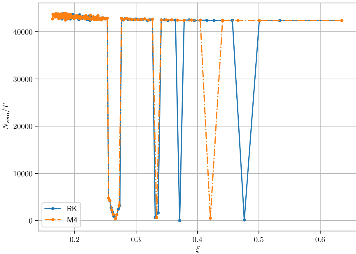
Число переходов нуля на квазипериод для \text{Re } \psi_2 , разные методы
