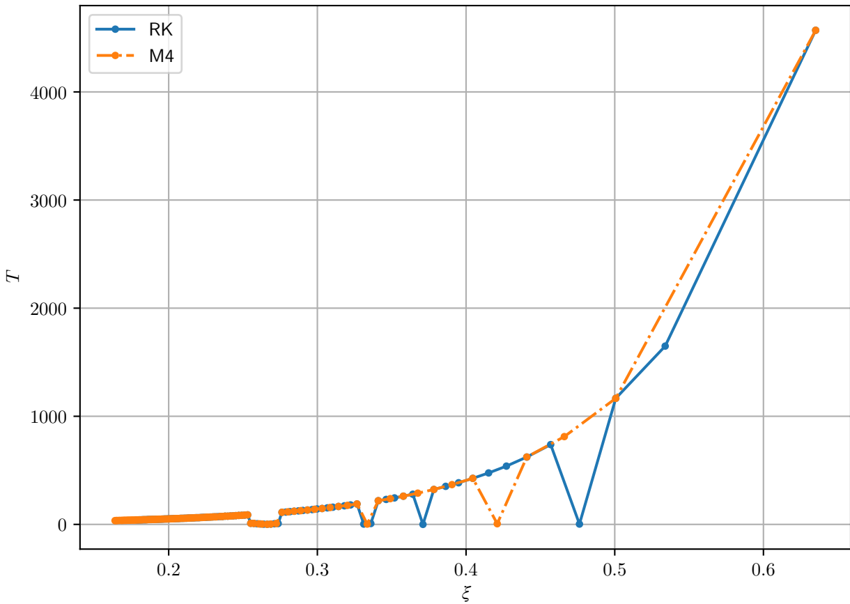
Квазипериод \text{Re } \psi_2 , разные методы
