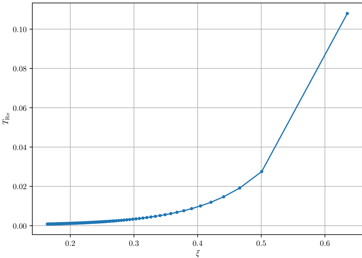
Квазипериод реальной части \phi_1
