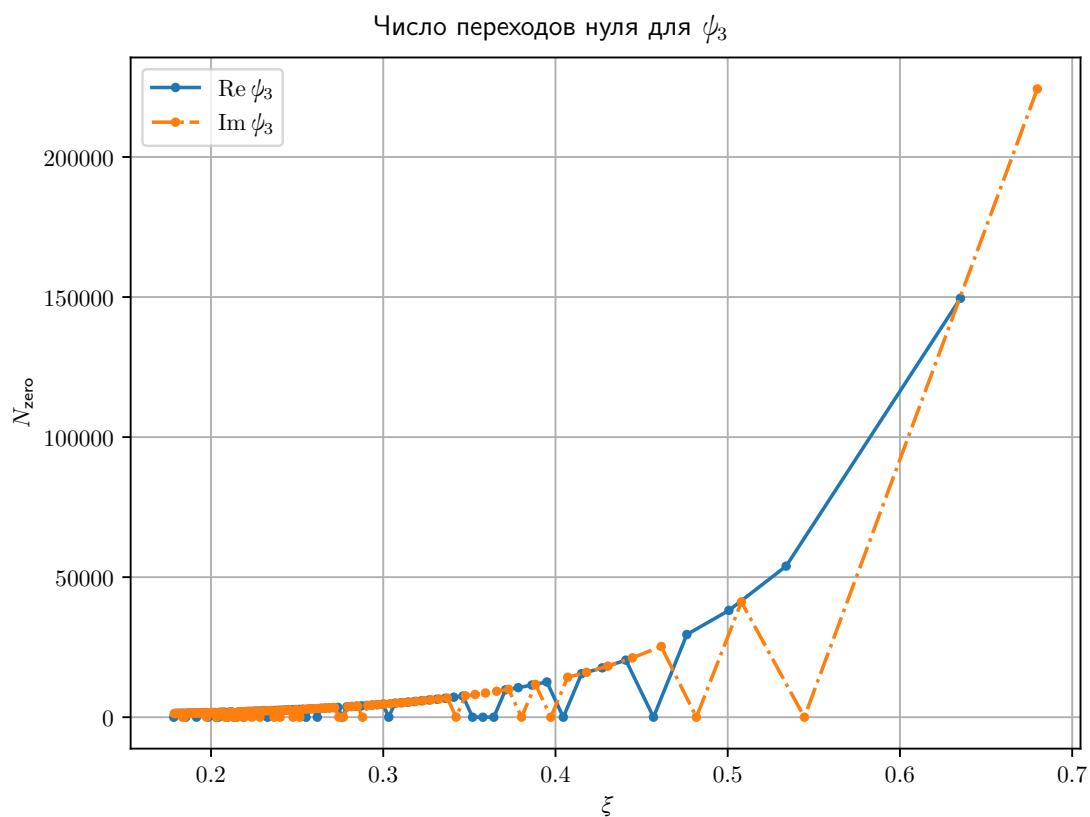
Рисунок 4 — График количества переходов через ноль Re \psi_3 и Im \psi_3 на интервале одного квази-периода \psi_1 по данным DOPRI
