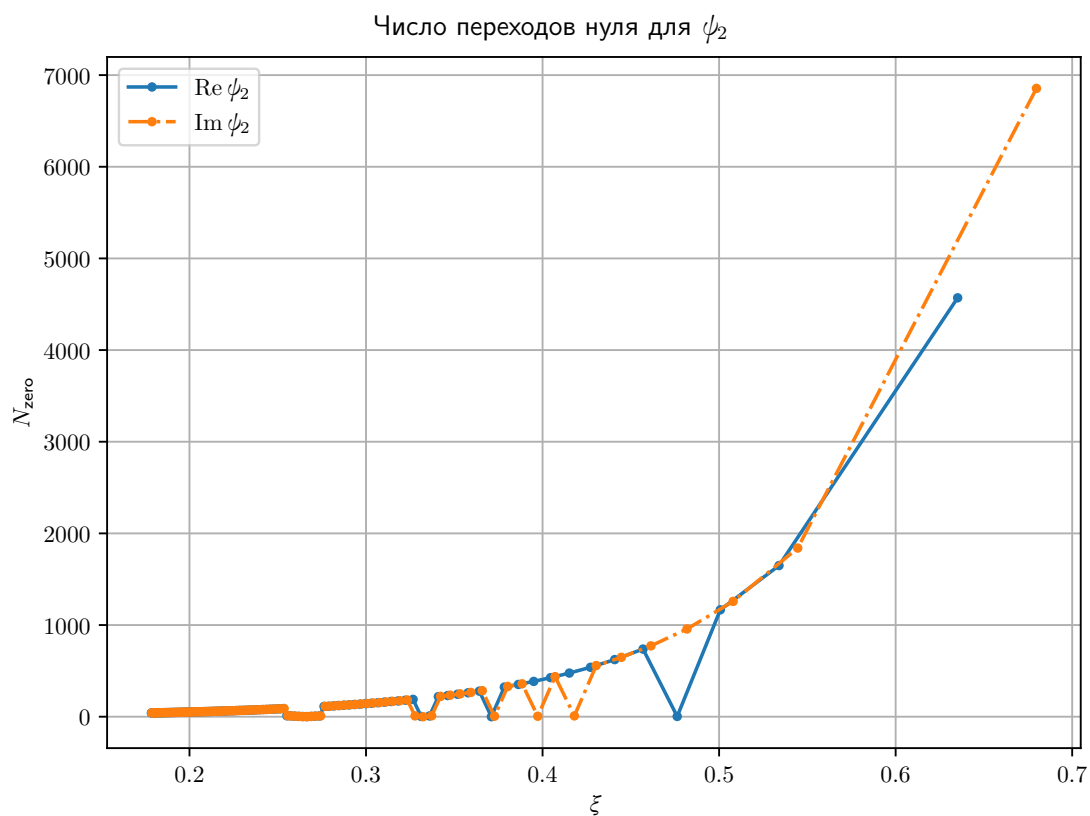
Рисунок 3 — График количества переходов через ноль Re \psi_2 и Im \psi_2 на интервале одного квази-периода \psi_1 по данным DOPRI
