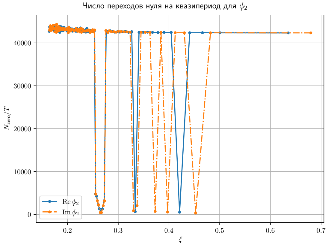
Рис. 13: График количество нулей \text{Re } \Psi_2 и \text{Im } \Psi_2 на единицу длины квазипериода \Psi_1 по данным М4
