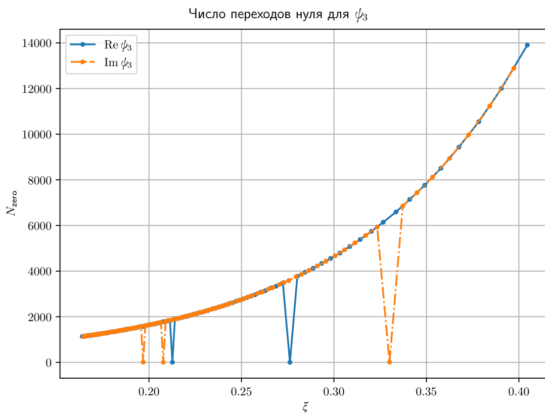
Рис. 12: График количества переходов через ноль \text{Re } \Psi_3 и \text{Im } \Psi_3 на интервале одного квазипериода \Psi_1 по данным М4
