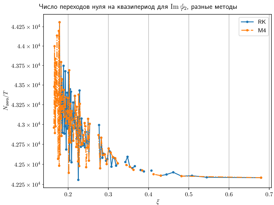
Рис. 21: График количество нулей \text{Im } \Psi_2 на единицу длины квазипериода \text{Im } \Psi_1 по данным M4 и DOPRI
