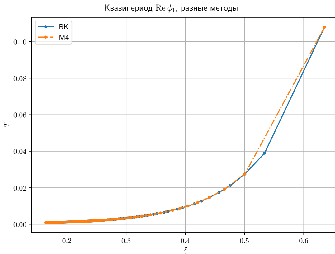
Рис. 17: График зависимости длины квазипериода \text{Re } \Psi_1 от \xi по данным M4 и DOPRI
