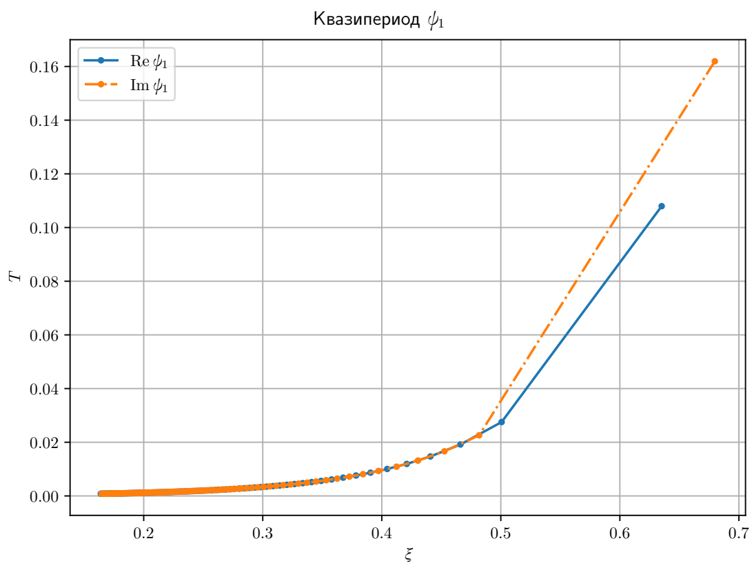
Рис. 10: График зависимости длины квазипериода \text{Re } \Psi_1 и \text{Im } \Psi_1 от \xi по данным М4
