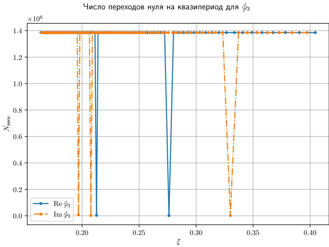
Рис. 14: График количество нулей \text{Re } \Psi_3 и \text{Im } \Psi_3 на единицу длины квазипериода \Psi_1 по данным М4
