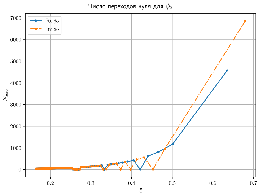
Рис. 11: График количества переходов через ноль \text{Re } \Psi_2 и \text{Im } \Psi_2 на интервале одного квазипериода \Psi_1 по данным М4
