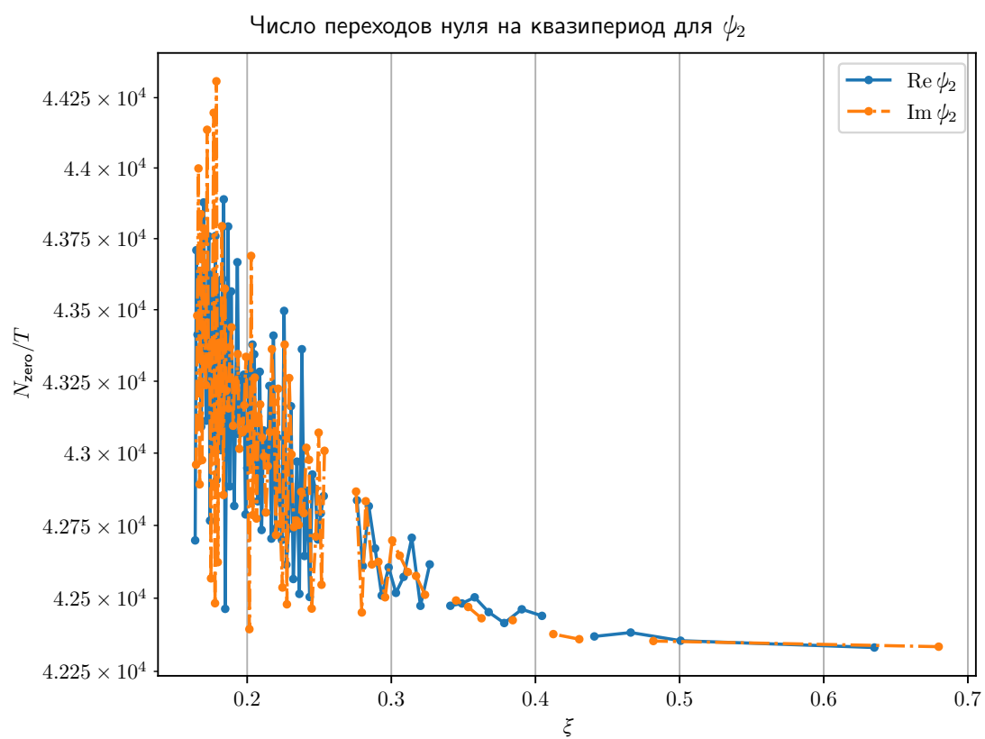
Рис. 15: График количество нулей Re\Psi_2 и Im\Psi_2 на единицу длины квазипериода \Psi_1 из данных DOPRI без выбросов
