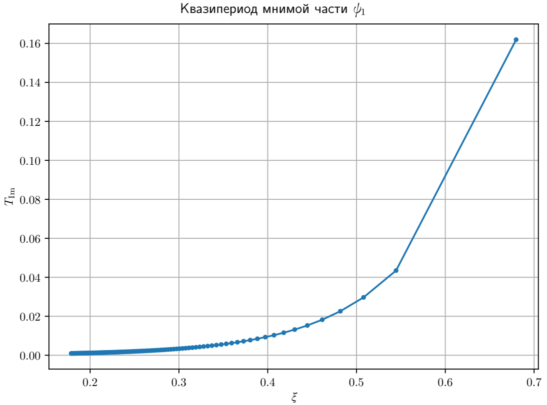
Рис. 4: График зависимости длины квазипериода Im\Psi_1 от \xi
