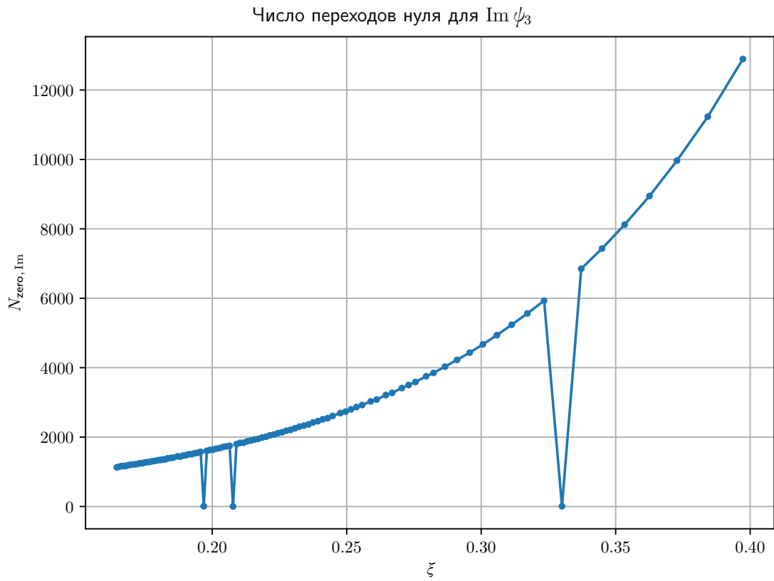
Рис. 18: График количества переходов через ноль \text{Im}\Psi_3 на интервале одного квазипериода \text{Im}\Psi_1 из данных magexr
