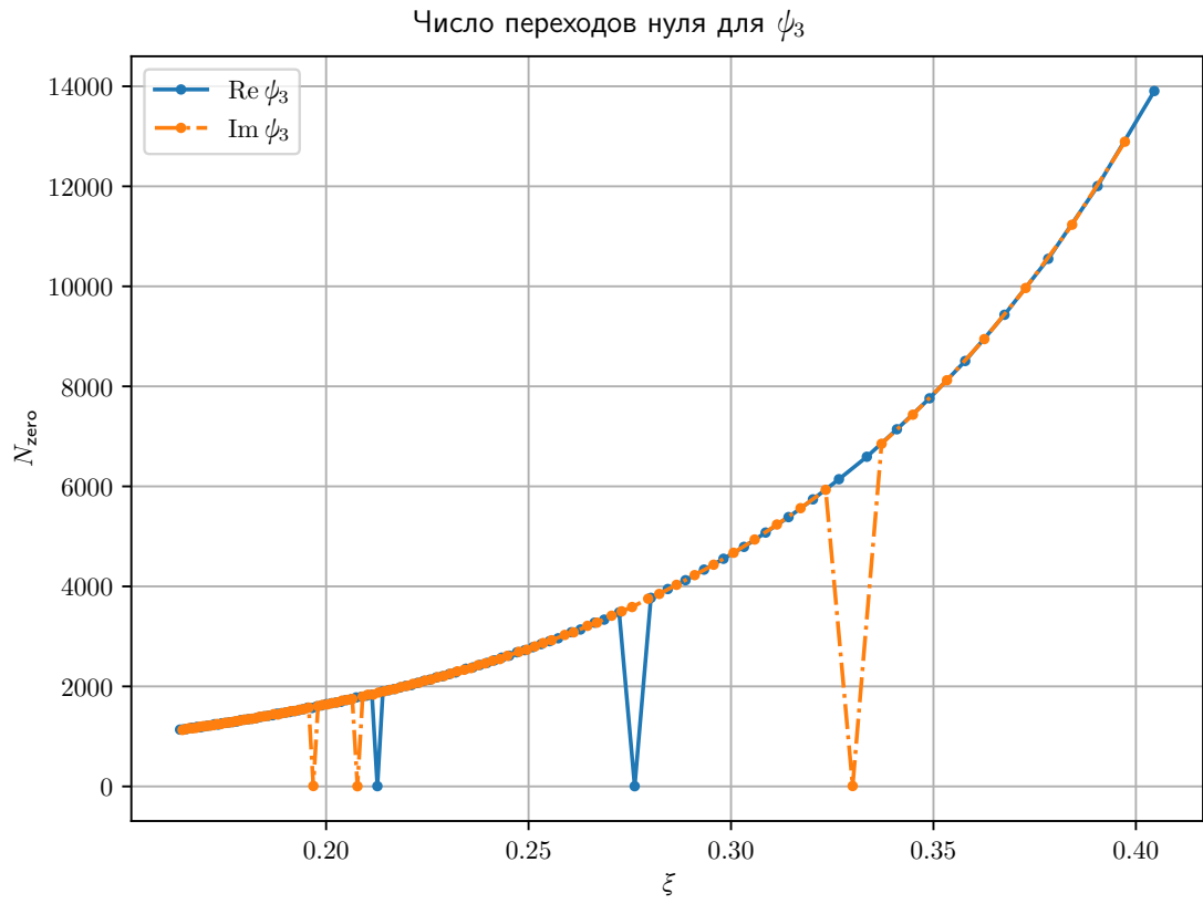
Рис. 12: График количества переходов через ноль \text{Re } \Psi_3 и \text{Im } \Psi_3 на интервале одного квазипериода \Psi_1 по данным М4
