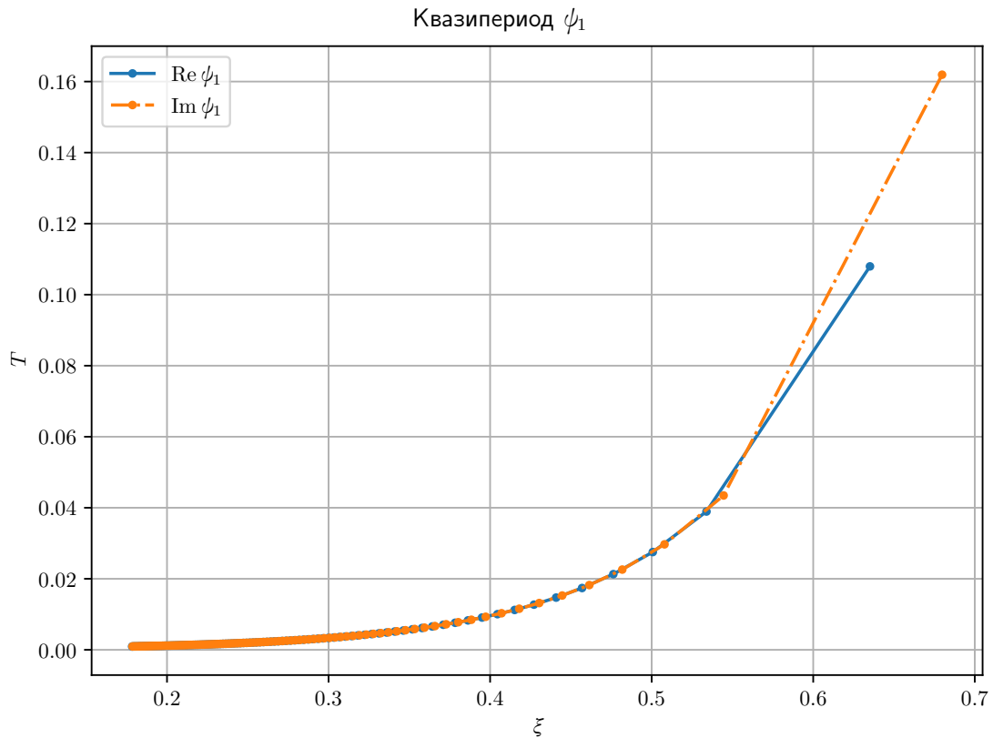
Рис. 2: График зависимости длины квазипериода Re\Psi_1 и Im\Psi_1 от \xi по данным DOPRI
