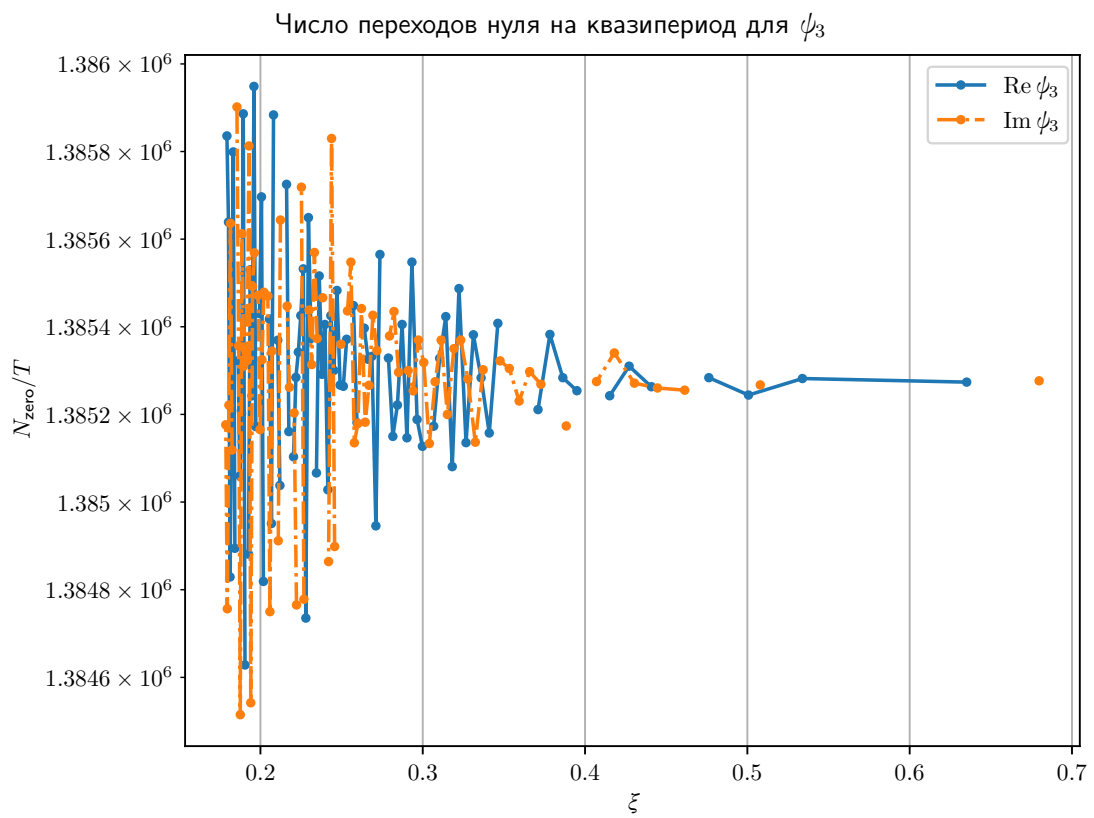
Рис. 9: График количество нулей \text{Re}\Psi_3 и \text{Im}\Psi_3 на единицу длины квазипериода \Psi_1 из данных DOPRI без выбросов
