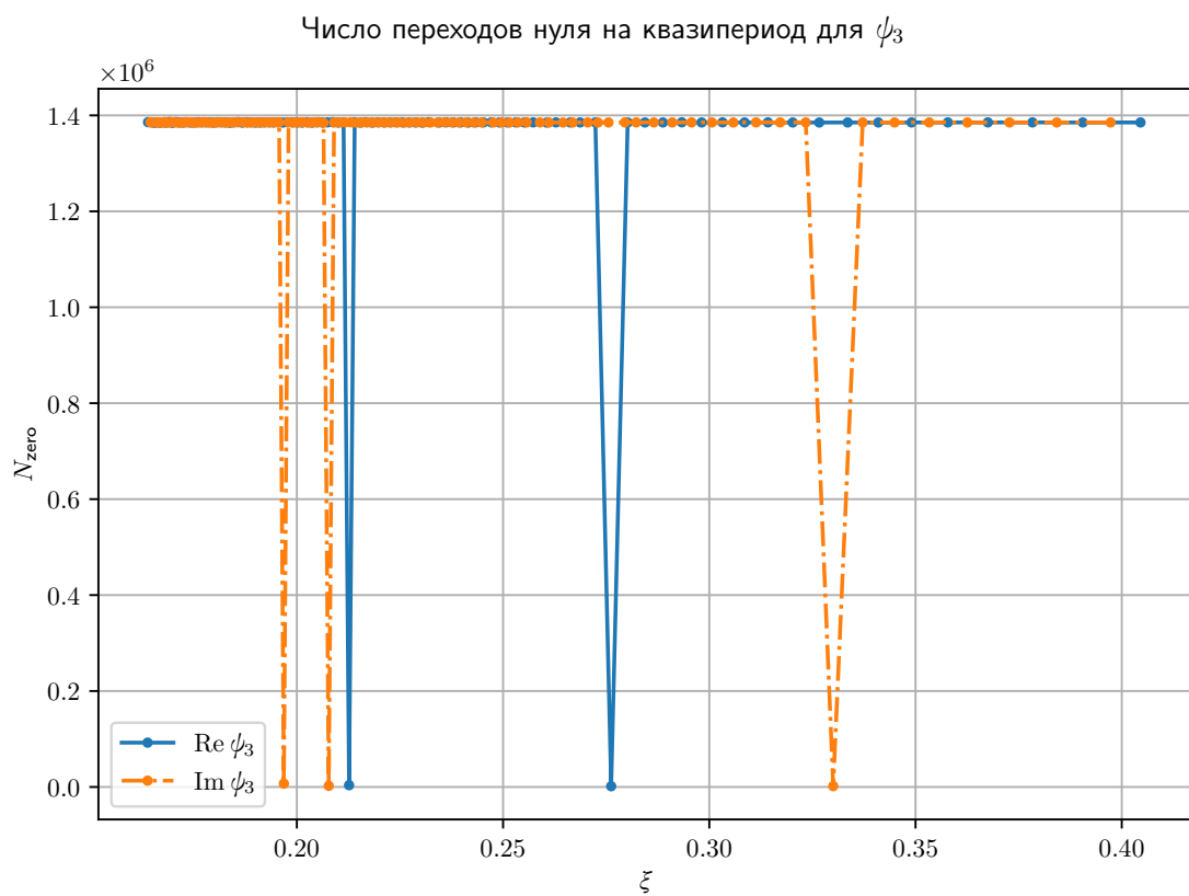
Рис. 14: График количество нулей Re\Psi_3 и Im\Psi_3 на единицу длины квазипериода \Psi_1 из данных М4
