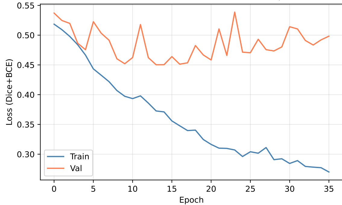
Courbes d'entraînement — DPT + ViT-B/16
