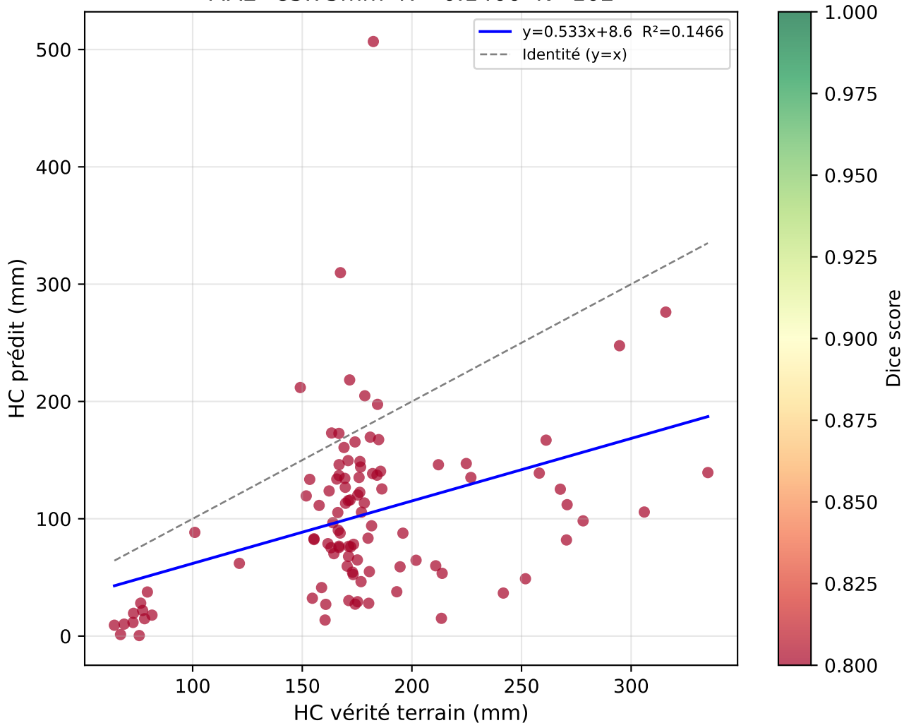
HC prédit vs GT — HC18 test MAE=85.75mm R^2=0.1466 N=102
