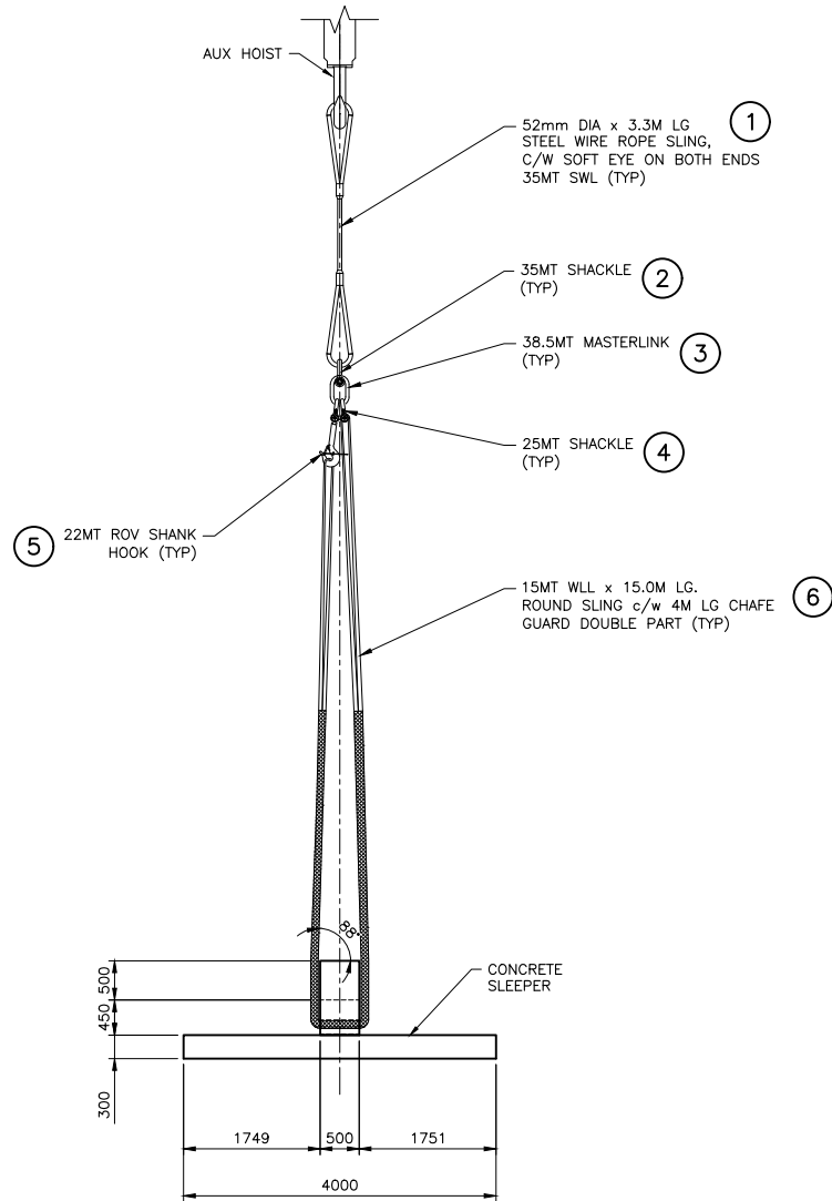
ELEVATION
