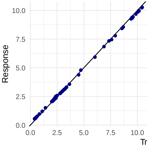
regr.cv_glmnet
