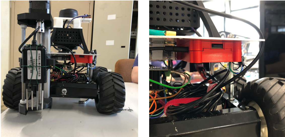
FIGURE 2 – Raspberry Pi fixé sous le châssis supérieur et câble USB-C.
