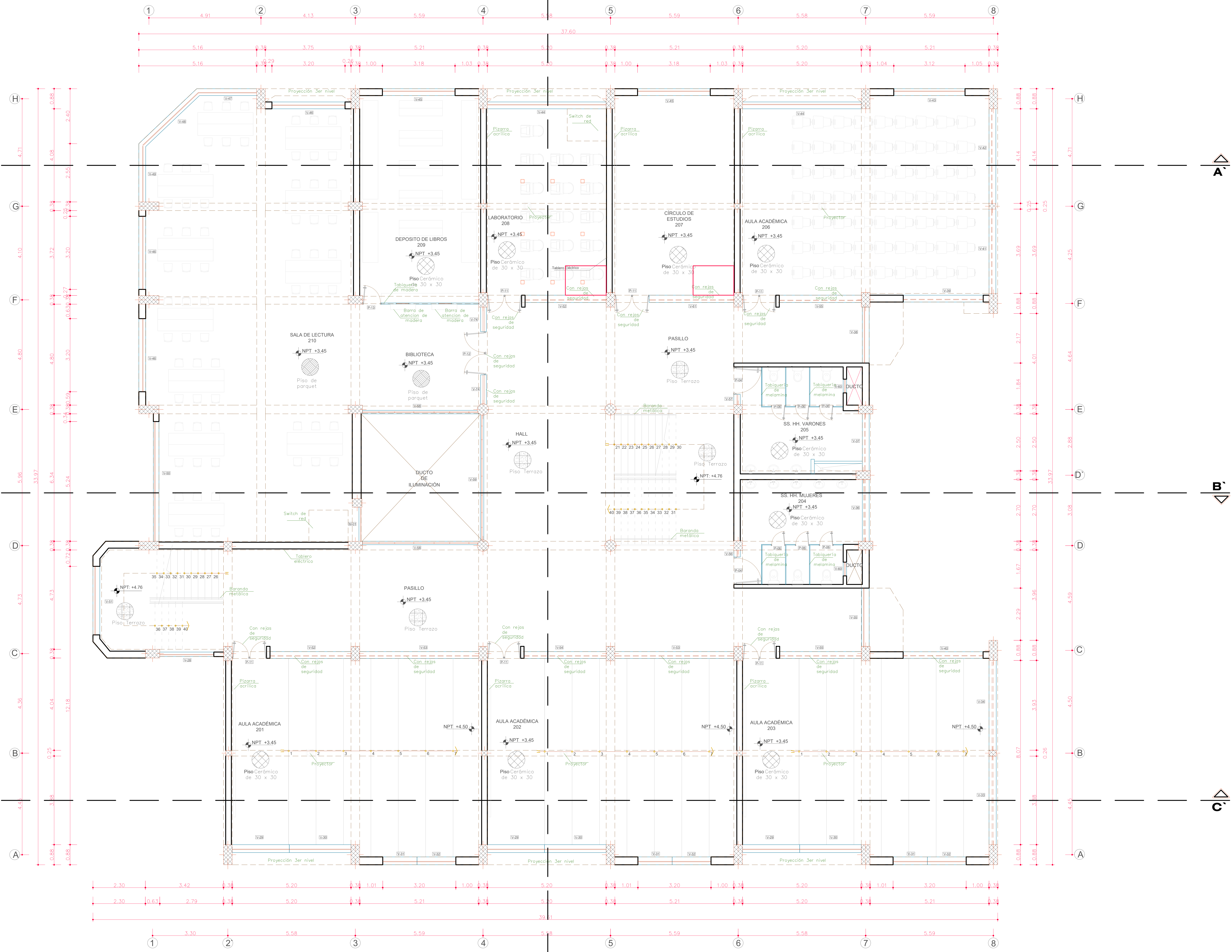
PLANO DE DISTRIBUCION SEGUNDO NIVEL
