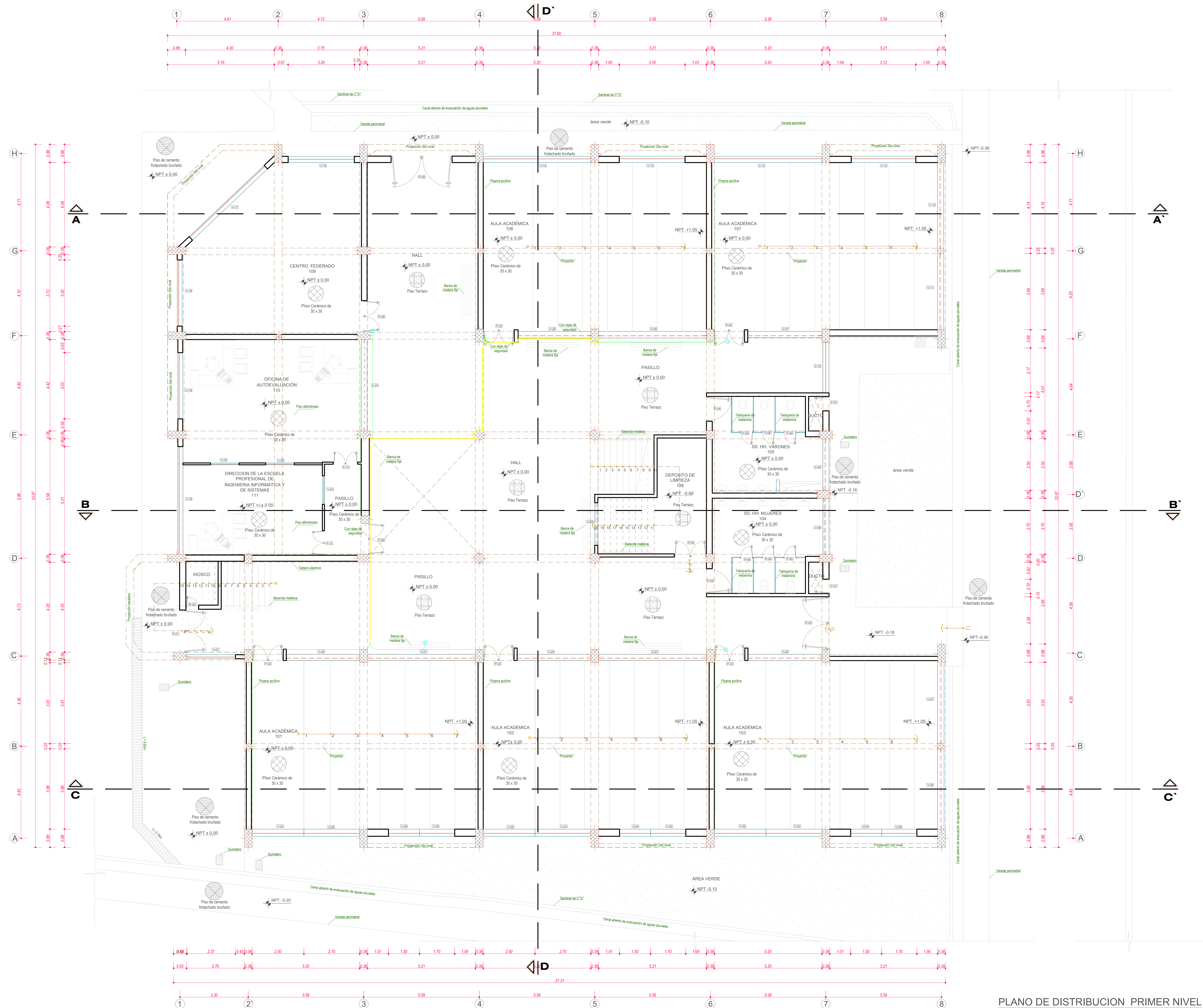
PLANO DE DISTRIBUCION PRIMER NIVEL ESC:1/75
