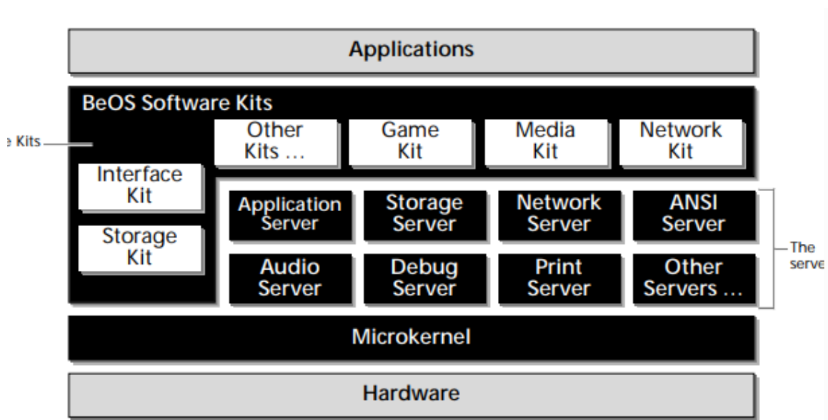
Figura 1.4: Arquitectura del sistema operativo BeOS.
