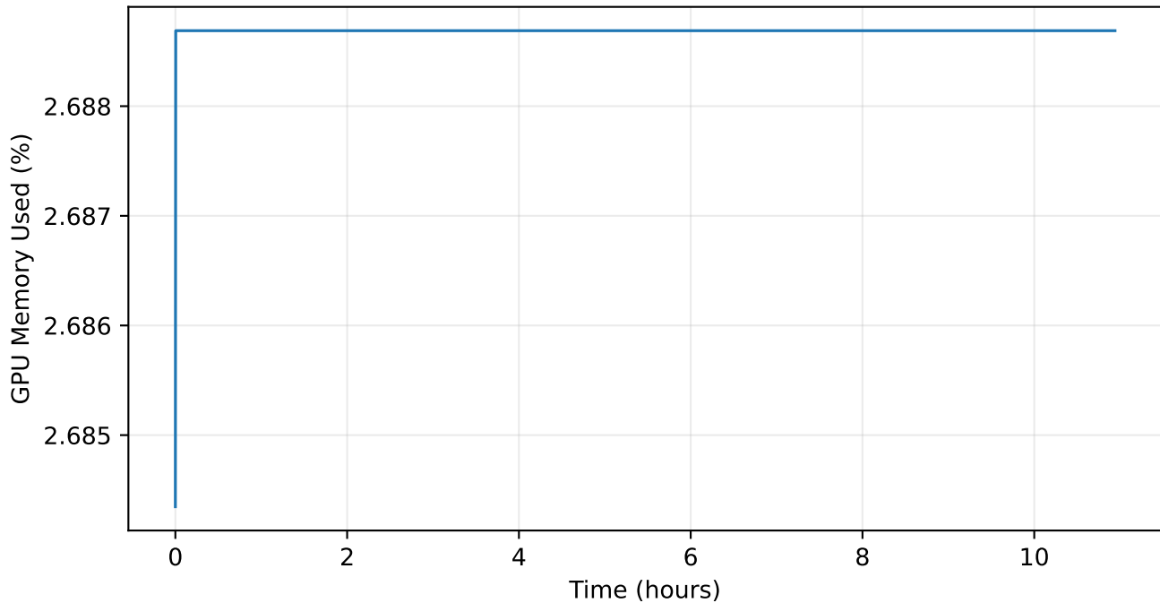
GPU Memory %
