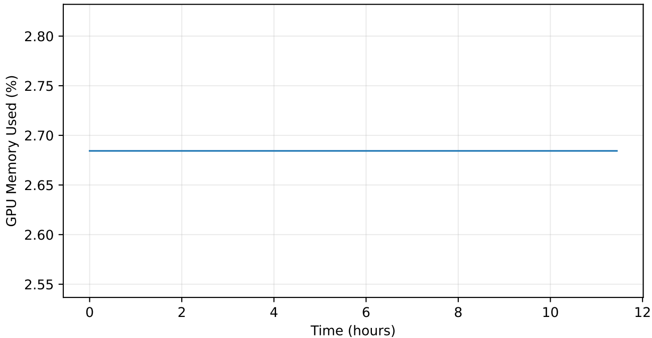
GPU Memory %
